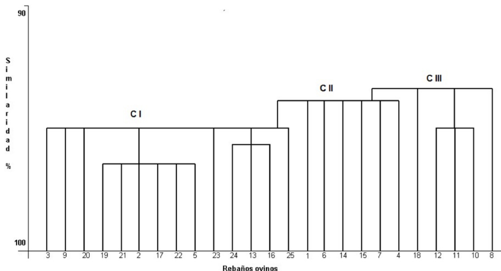
Figura 1. Diagrama de árbol de clasificación por similitud de los rebaños ovinos del sur de la Ciudad de México.
