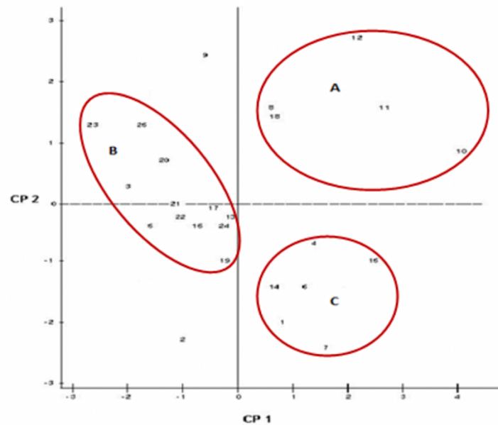
Figura 2. Dispersión de las unidades de producción ovina del sur de la Ciudad de México. Fuente: Elaboración propia.
