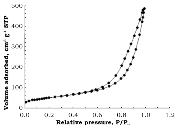
Figura 2. Isotherma de adsorción-desorción de N_2 a 77 K sobre HDL.
