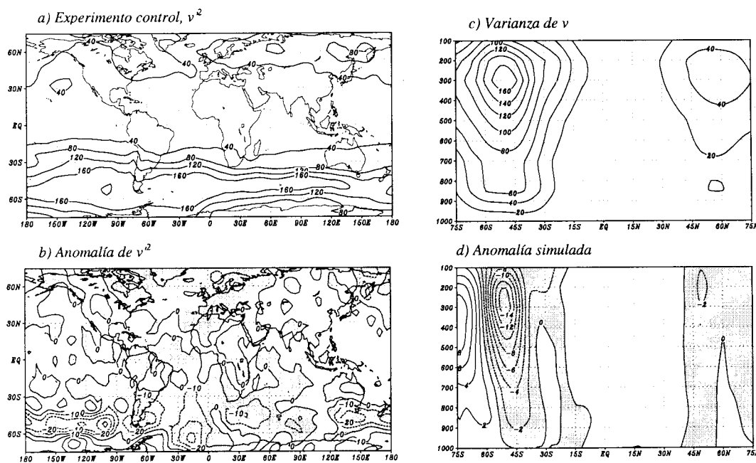
Fig. 4. Variabilidad de la componente meridional del viento en 300 hPa a) control (cada 40 m 2 /s 2 ), y b) anomalía (cada 10 m 2 /s 2 ). La variabilidad de v en promedio zonal c) control (cada 20 m 2 /s 2 ) y d) anomalía (cada 1 m 2 /s 2 ).
