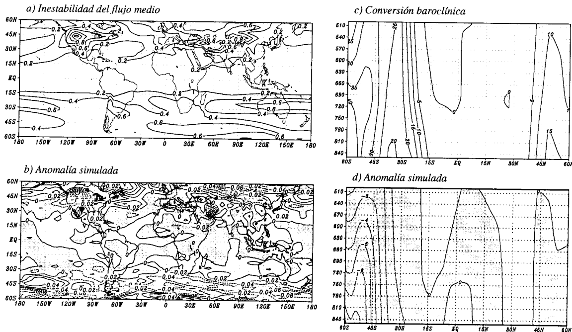
Fig. 3. A la derecha, se presenta la tasa de crecimiento de Eady: a) control (isolíneas cada 0.1/día) y b) diferencia entre el experimento A964911 y el control (cada 0.02/día). A la izquierda se muestra el término de conversión baroclínica promediado zonalmente: c) control (cada 5 m 2 /s 2 /día) y d) anomalía simulada (2 m 2 /s 2 /día). Para b) y d) se sombreadon las regiones con valores negativos.
