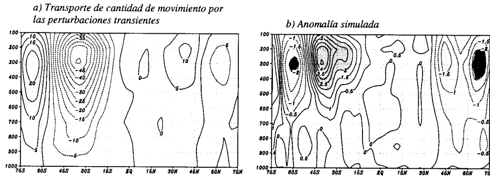
Fig. 6. Promedio zonal del transporte de cantidad de movimiento por las perturbaciones transitorias: a) experimento control (cada 5 \text{ m}^2/\text{s}^2 ) y b) anomalía simulada (cada 0.5 \text{ m}^2/\text{s}^2 ). Las regiones sombreadas destacan las anomalías superiores a 2 \text{ m}^2/\text{s}^2 (en valor absoluto).
