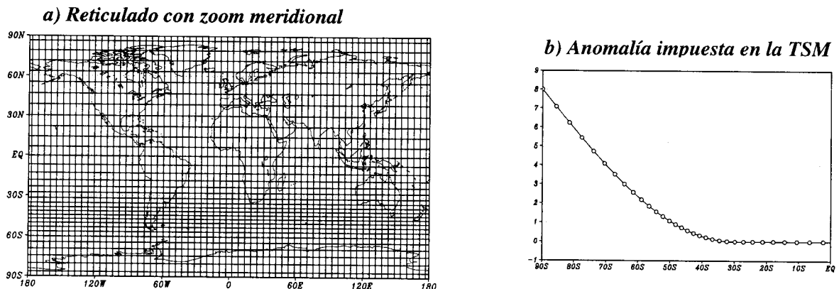
Fig. 1. a) Reticulado definido para las experiencias realizadas; b) anomalía adicionada a los campos climatológicos de la TSM, en el experimento A964911.
