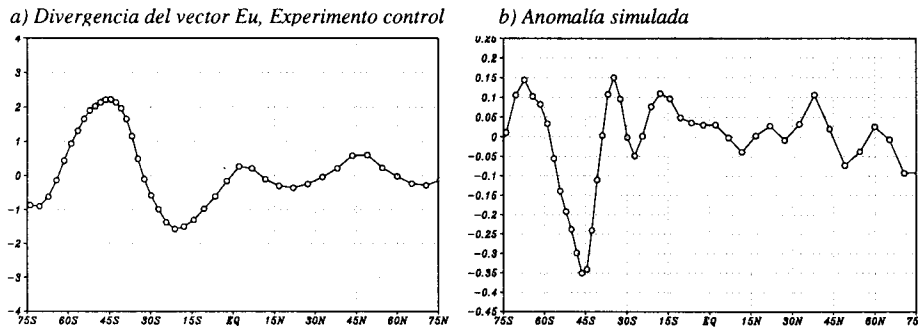
Fig. 7. Divergencia del vector E_u en promedio zonal. a) experimento de control, b) anomalía simulada.
