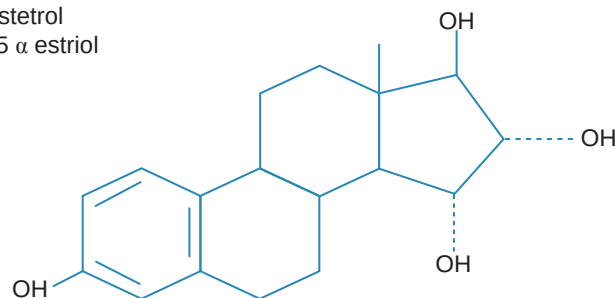
Figura 2: Estructura molecular del estetrol (E4) 5α-hidroxiestradiol; Estra-1,3,5(10)-triene-3,15α,16α,17β-tetrol.
