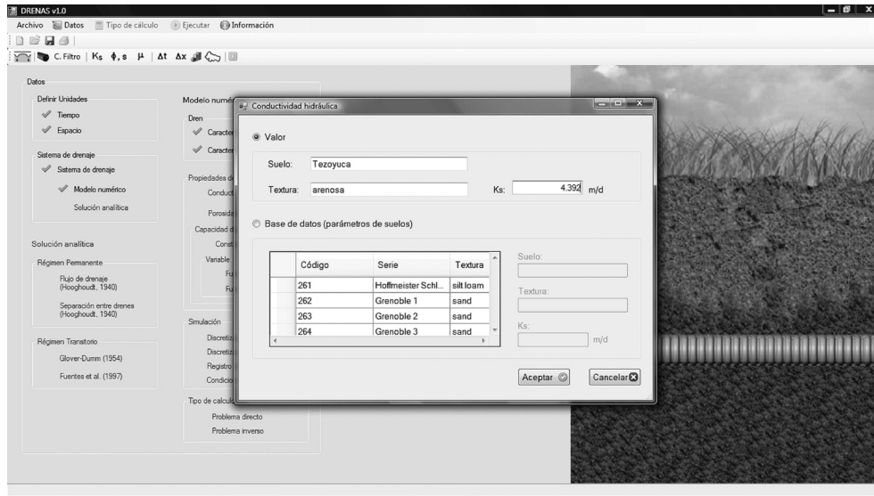
Figura 4. Ingreso de parámetros del suelo: a) directa; o b) base de datos.
