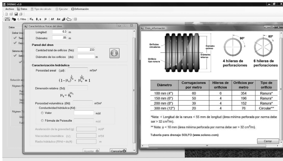
Figura 5. Definición de datos de los drenes con información de soporte.
