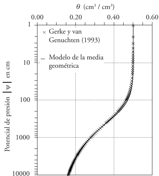
A) Modelo del poro geométrico, ecuación 11 sujeta a sm=1-2s/n , para m=0.29 y \psi_d=-195 cm (RECM=0.004 cm 3 /cm 3 ).
