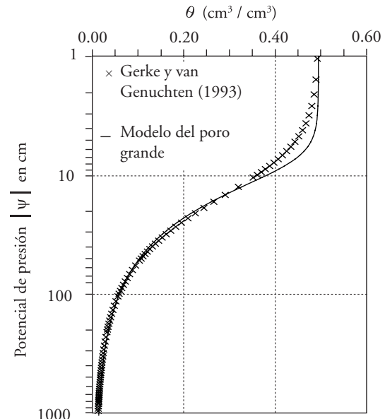
B) Modelo del poro grande, ecuación 11 sujeta a 2sm=1-4s/n , para m=0.223 y \psi_d=-7.8 cm (RECM=0.009 cm 3 /cm 3 ).
