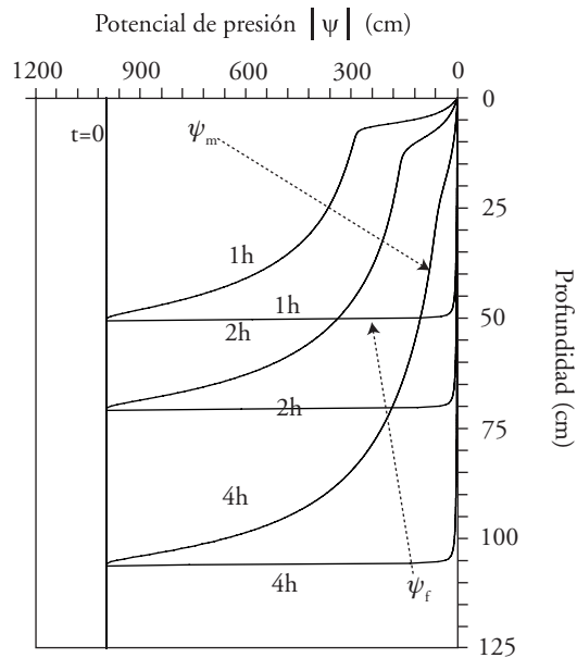
Figura 6. Distribución del potencial de presión del agua en la matriz (m) y el macroporo (f).
