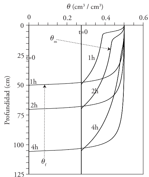
Figura 8. Distribución del contenido volumétrico de agua en la matriz (m) y el macroporo (f).
