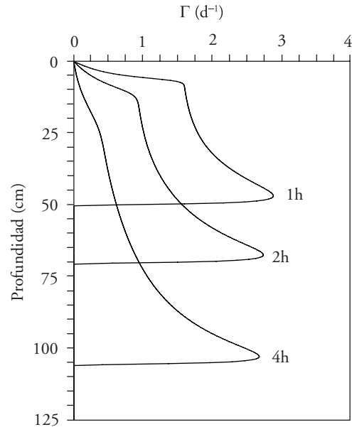
Figura 7. Distribución de la tasa de transferencia de agua ( \Gamma_w ) en diferentes tiempos.
