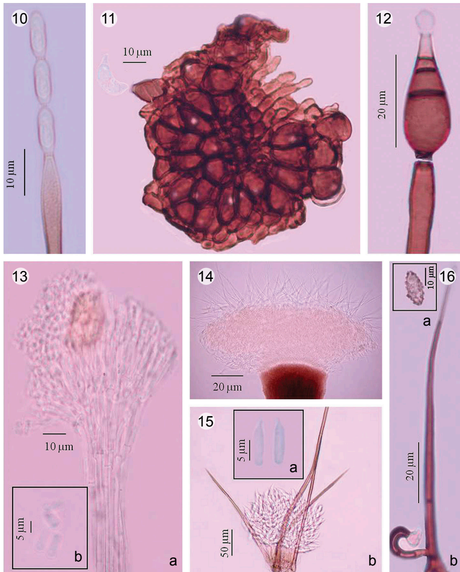
Figs. 10-16. 10. Monilochaetes guadalcanalensis : conidióforo con conidios catenulados. 11. Mycoleptodiscus taiwanensis : esporodocio y conidio. 12. Sporidesmium dissolvens : conidióforo con conidio obclavado con gota mucilaginosa en el ápice. 13. Stilbella clavispora : a. parte apical del sinema con células conidiógenas y conidios, b. conidios claviformes. 14. Thozetella havanensis : sinema con aristas y conidios. 15. Vermiculariopsiella parvula : a. conidios, b. esporodocio con setas y conidios. 16. Zygosporium geminatum : a. conidio elipsoidal verrugoso, b. conidióforo con vesícula y célula conidiógena integrada.
