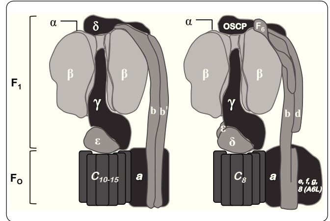
Figura 1. Organización polipeptídica de las F 1 F o -ATP sintasas. Las F-ATPasas bacterianas y cloroplastídicas se muestran a la izquierda, mientras que la mitocondrial se encuentra a la derecha. La parte superior de cada modelo contiene a las subunidades catalíticas ( \alpha_3\beta_3 ) del dominio F 1 . Una de las tres subunidades \alpha ha sido removida para exponer a la subunidad \gamma , cabe resaltar que ésta abarca desde el eje central del dominio catalítico hasta el anillo de subunidad c y la subunidad a . De igual forma, el brazo periférico de cada modelo se muestra a la derecha. En algunas bacterias está compuesto por la subunidad \delta y el dímero de subunidad b . Mientras que en otras especies bacterianas, así como en la enzima cloroplastídica, las dos subunidades b son copias homólogas, pero no idénticas (subunidad b y b' ). En la enzima mitocondrial, el brazo periférico lo componen una copia de las subunidades b , d y F 6 . El dominio membranal de la enzima mitocondrial contiene subunidades con una hélice transmembranal ( e , f , g , 8 (A6L), entre otras descritas en la Tabla I), las cuales no se encuentran en las ATPasas bacterianas y cloroplastídicas. Modificado de Walker, 2013.
