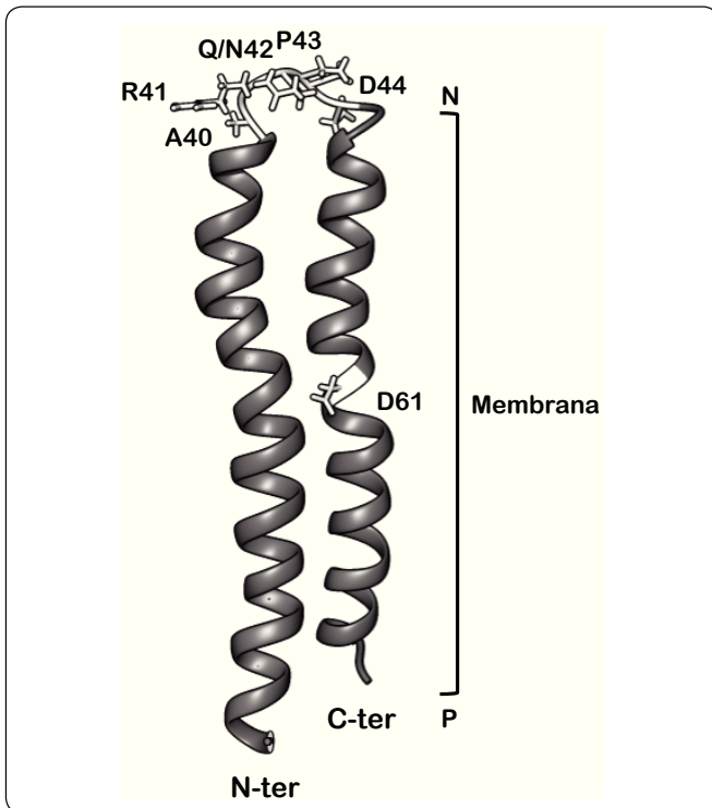
Figura 5. Representación de la estructura tipo horquilla de la subunidad c bacteriana sugerido por estudios de RMN a pH 5. Se indica la orientación de la estructura en la membrana, lado positivo (P) y lado negativo (N), así como del extremo amino (N-ter, proyectado al frente) y carboxilo terminal (C-ter, proyectado hacia el fondo). Asimismo, se muestran las posiciones de los residuos clave discutidos en el texto. Las coordenadas PDB de la estructura son 1C0V. Modificada de Girvin et al. , 1998; Fillingame & Dmitriev, 2002.
