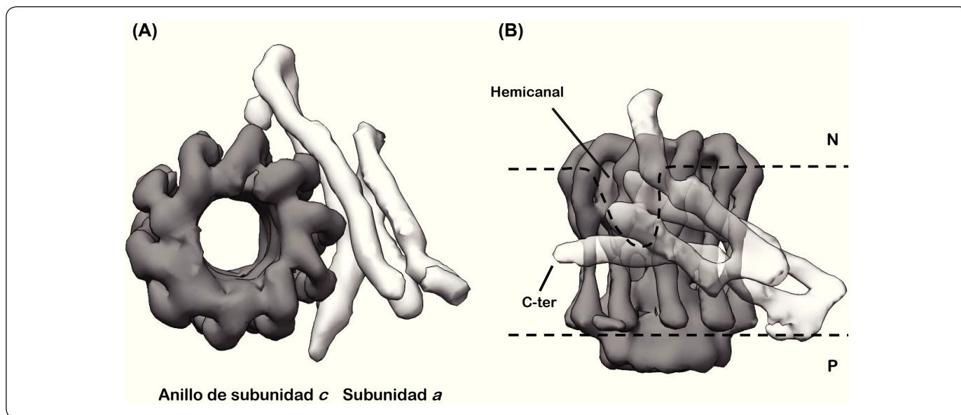
Figura 10. Modelo estructural del anillo de subunidades c-subunidad a. (A) Imágenes obtenidas por crío-microscopía electrónica (7.0 Å de resolución, no. de acceso EMD 2852) de un corte transversal a nivel de membrana del dominio F_0 de la ATP sintasa de Polytomella sp., en donde se muestra a la izquierda el anillo de subunidad c (negro) y a la derecha la densidad electrónica de las hélices horizontales membranales de la subunidad a (gris). En este modelo no se representa al amino terminal. (B) Vista lateral de (A), en donde se muestra al anillo de subunidad c al fondo (negro), y hacia el frente los segmentos alfa-helicoidales atravesando la membrana de manera horizontal (cuatro segmentos en gris). Se señala tanto el hemicanal formado por la interacción de ambas subunidades, así como la región carboxilo (C-ter) de la subunidad a. P = lado positivo, N = lado negativo. Modificado de Allegretti et al., 2015; Kühlbrandt & Davies, 2016.
