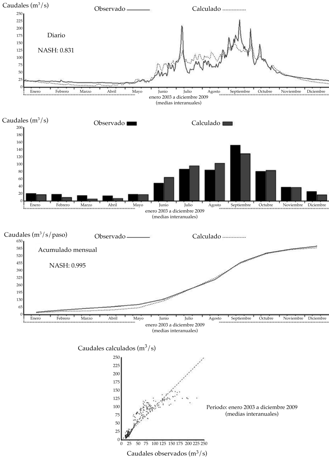
Figura 4. Histogramas e hidrogramas con EMA.
