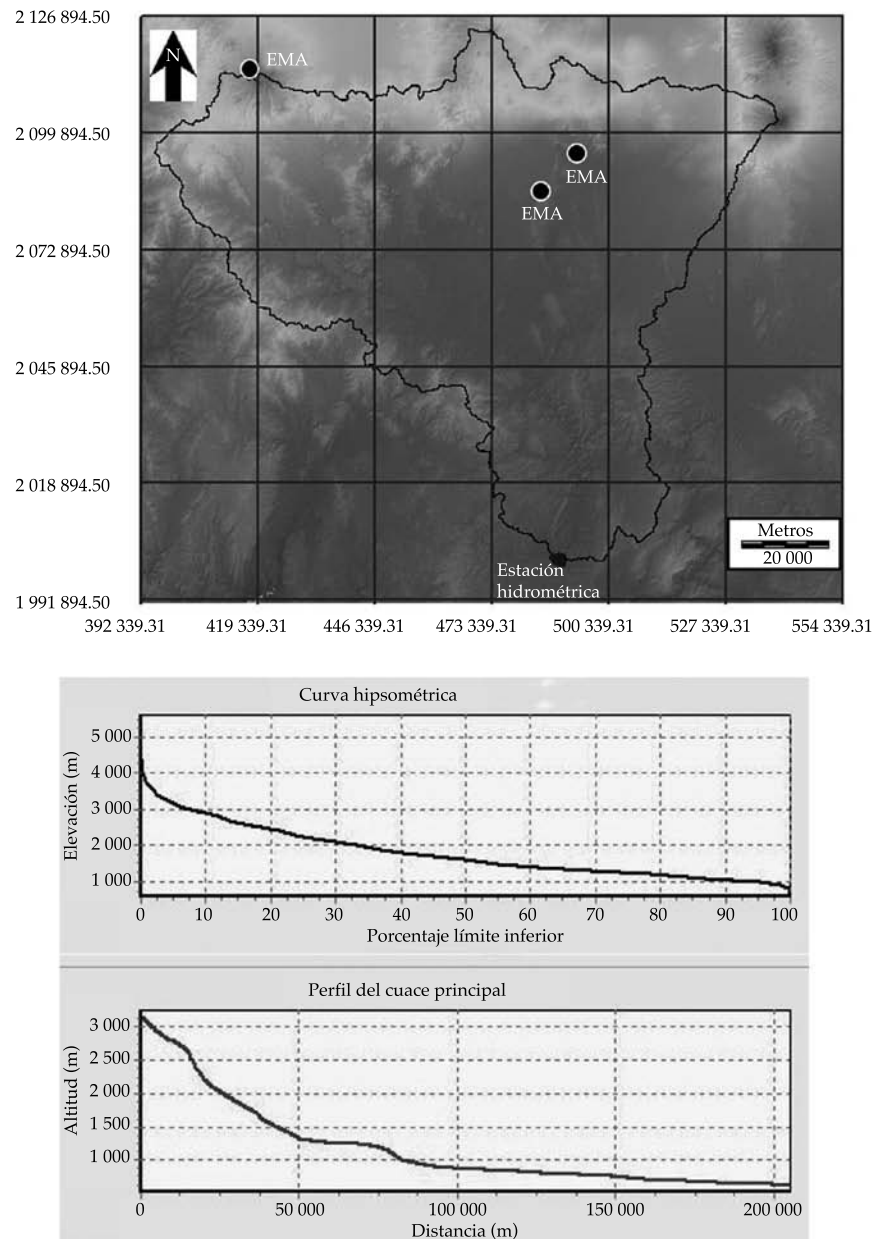
Figura 2. Delimitación, ubicación de EMA, curva hipsométrica y perfil de la cuenca hasta la estación hidrométrica Atenango del Río.
