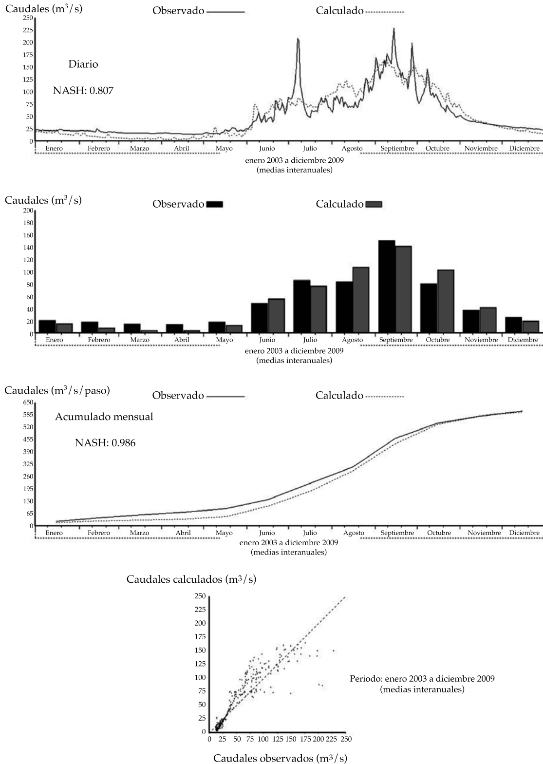
Figura 6. Histogramas e hidrogramas con imágenes PERSIANN (interanuales, 2003-2009).
