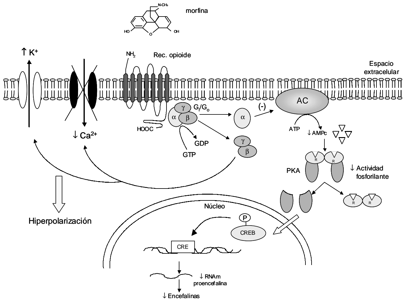
Fig. 1. Efectos inhibitorios agudos de los opioides. Los agonistas opioides interactúan con receptores acoplados a una proteína G inhibitoria (G i /G o ), la cual se disocia en la subunidad α y el complejo βγ. Por medio de la subunidad α se inhibe la adenilato ciclasa (AC), con lo cual disminuye la formación de AMPc (triángulos). Este segundo mensajero activa la proteína cinasa dependiente de AMPc (PKA) al unirse a las subunidades regulatorias (R) y liberar a las catalíticas, las cuales fosforilan a diversas proteínas. Entre éstas, la proteína CREB fosforilada ( cAMP response element binding protein ) actúa como factor de transcripción ya que se une a una región promotora del DNA llamada CRE y regula la síntesis de varias proteínas, incluida la de los péptidos opioides. Asimismo, los agonistas opioides activan los canales rectificadores entrantes de K + e inhiben los canales de Ca 2+ sensibles a voltaje a través del complejo βγ de la proteína G i . Estos efectos se traducen en una hiperpolarización celular. Modificado de Feldman (10).
