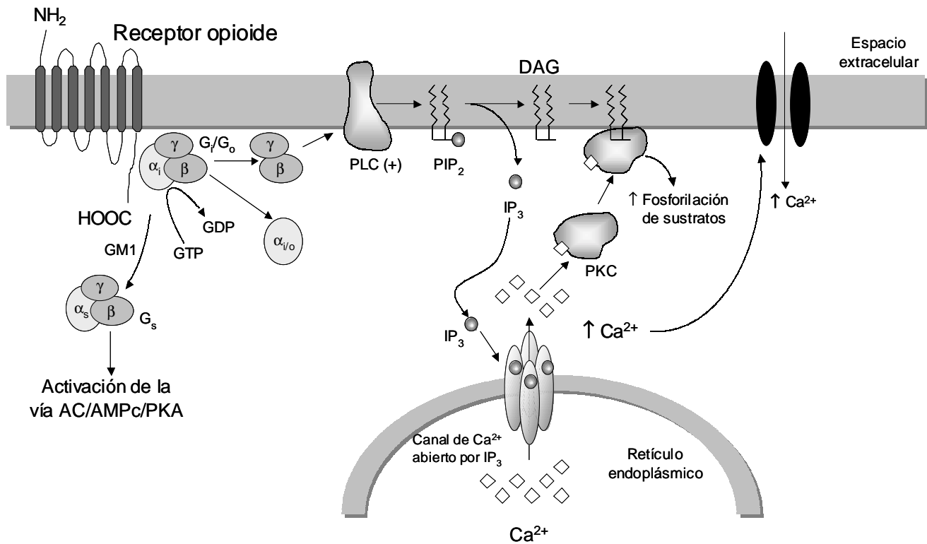
Fig. 2. Efectos estimulatorios de los opioides. El complejo βγ de la proteína G activa la fosfolipasa C (PLC), la cual convierte el lípido membranal fosfatidil-inositol (PIP 2 ) en dos derivados: el trifosfato de inositol (IP 3 ) y el diacilglicerol (DAG). El DAG permanece en la membrana, mientras que el IP 3 difunde el citosol y se une a canales de Ca 2+ del retículo endoplásmico para activarlos, lo que permite la salida de Ca 2+ (rombos) al citoplasma. Este catión se une a la proteína cinasa C (PKC), la cual se trasloca a la membrana donde se une al DAG para activarse y fosforilar a diferentes sustratos, entre ellos, la propia PLC. Esta vía se densibiliza muy rápidamente en condiciones normales. Los receptores opioides también pueden acoplarse a una proteína G estimuladora (G s ) en lugar de a una proteína G i/o cuando están en presencia del gangliósido GM1. Adaptado de Crain y Shen (8) y Waldhoer (51).
