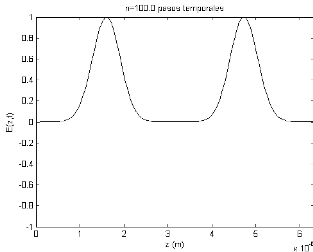
FIGURA 3. Pulso gaussiano después de 100 pasos temporales.
