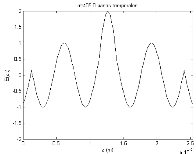
FIGURA 7. Superposición de dos ondas sinusoidales.
