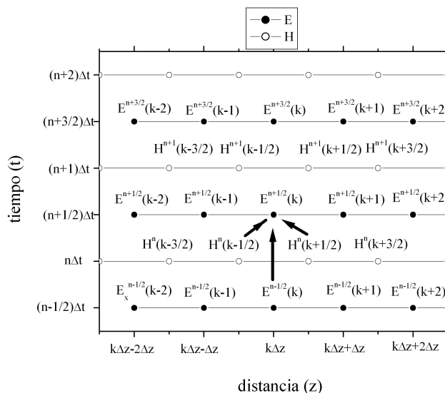
FIGURA 1. Representación de la evolución espacio-temporal de un campo electromagnético.
