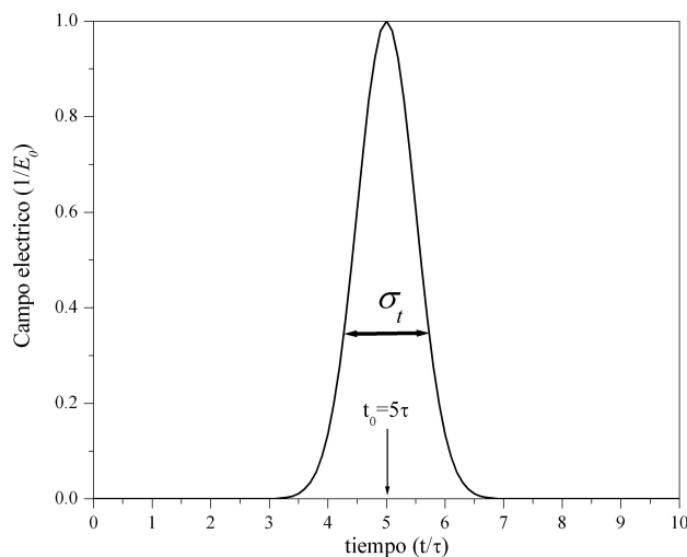
FIGURA 2. Ilustración de un pulso gaussiano, cuyo centro está en t = 5\tau y tiene un espesor \sigma_\tau .
