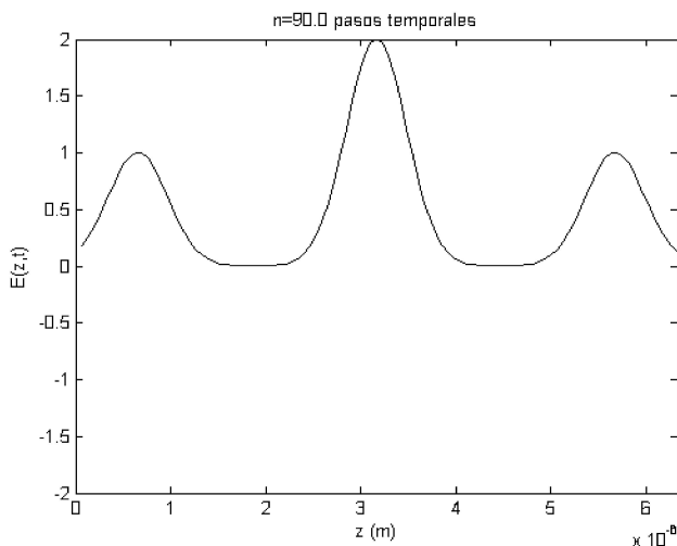
FIGURA 6. Superposición de dos pulsos gaussianos.
