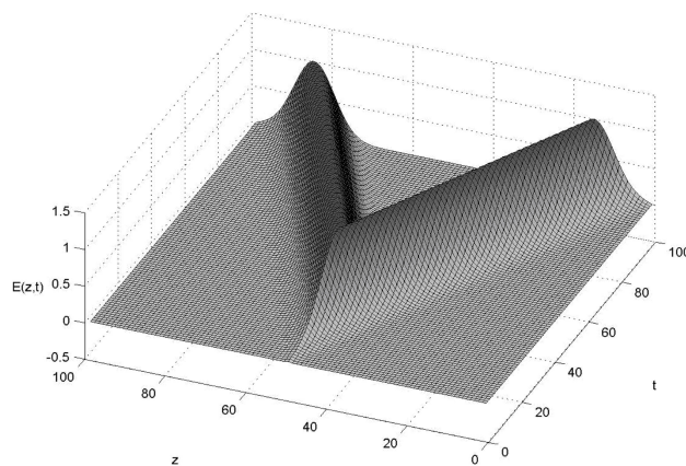
FIGURA 4. Variación del pulso gaussiano en el espacio y en el tiempo.
