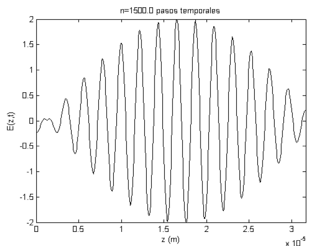
FIGURA 8. Evolución de la suma de dos ondas sinusoidales ligeramente desfasadas.
