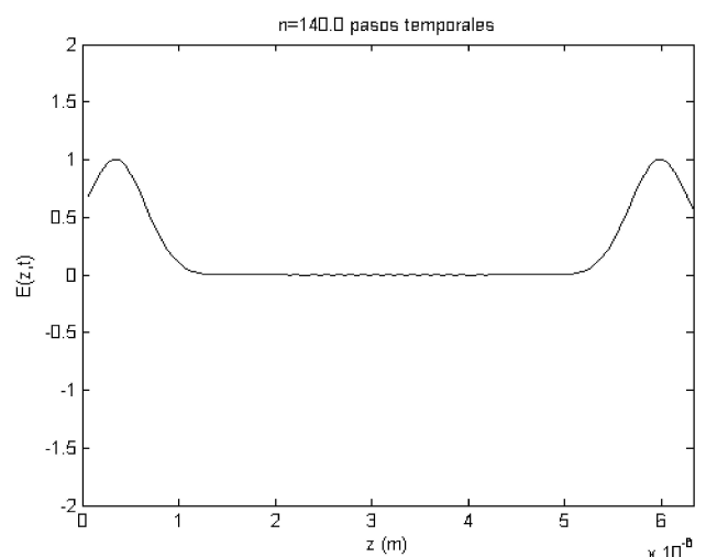
FIGURA 5. Pulso gaussiano después de 140 pasos temporales incluyendo condiciones absorbentes de frontera.
