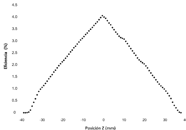
FIGURA 4. Eficiencia de la cámara en función del plano transversal del campo de visión.
