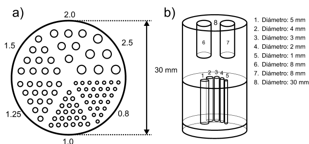
FIGURA 2. a) maniquí Derenzo en miniatura, b) maniquí de calidad de imagen tipo NEMA.
