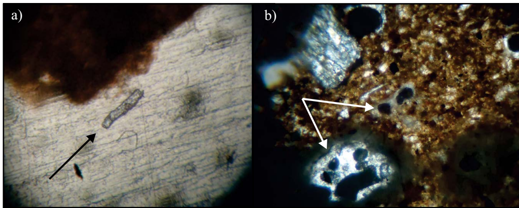
Figura 6. Componentes orgánicos en diferentes muestras de la facies 2. a) Fitolito elongito ( \times 10-100 \mu\text{m} a nicoles paralelos); b) fecas ( \times 10-100 \mu\text{m} a nicoles cruzados).
