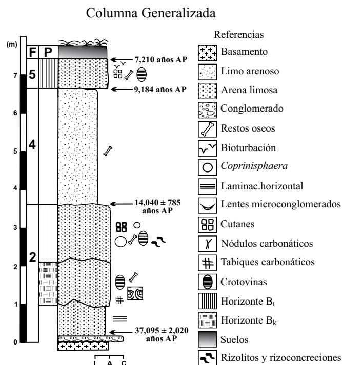
Figura 12. Columna Generalizada de la Fm. Vaca Corral (Krapovickas y Tauber, nueva Formación). F: facies; P: horizontes pedogenéticos inferidos.
