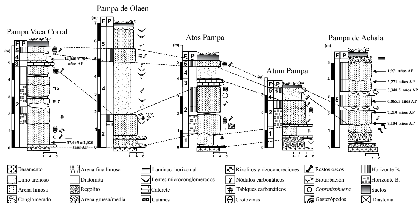
Figura 11. Perfiles estratigráficos generales de las localidades estudiadas, con la correlación geocronológica, lito y pedoestratigráfica. F: facies; P: horizontes pedogenéticos inferidos.
