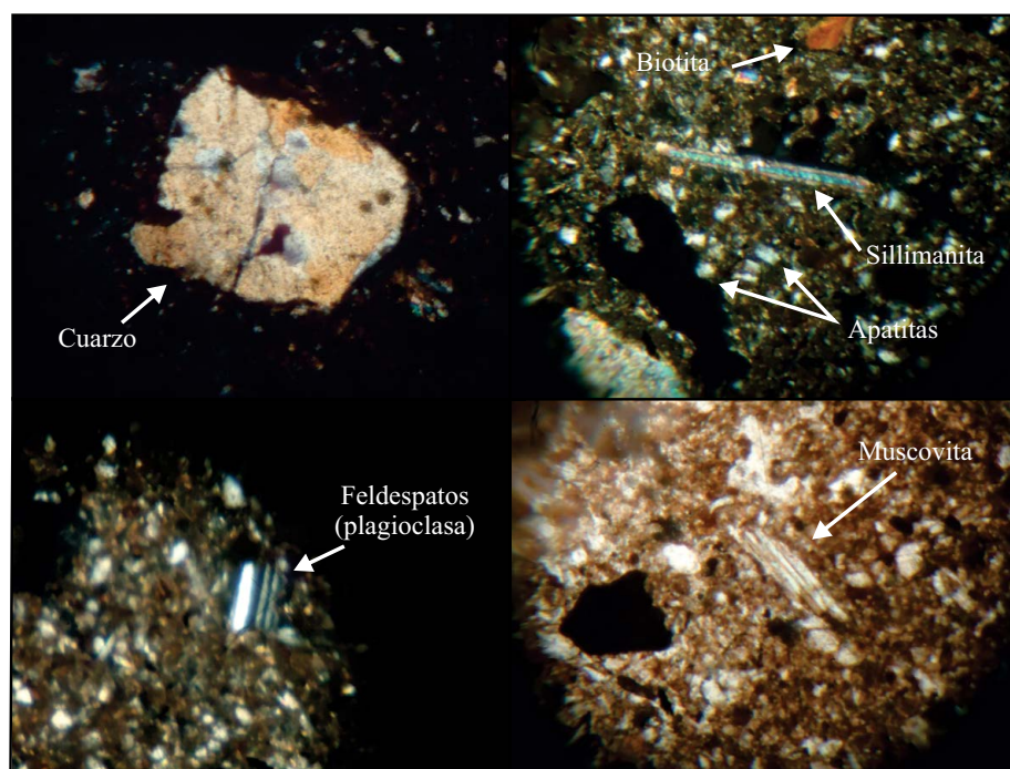
Figura 5. Principales componentes inorgánicos hallados en los estudios de microestructura realizados en diferentes muestras de la facies 2 ( \times 10-100 \mu\text{m} a nicoles cruzados).
