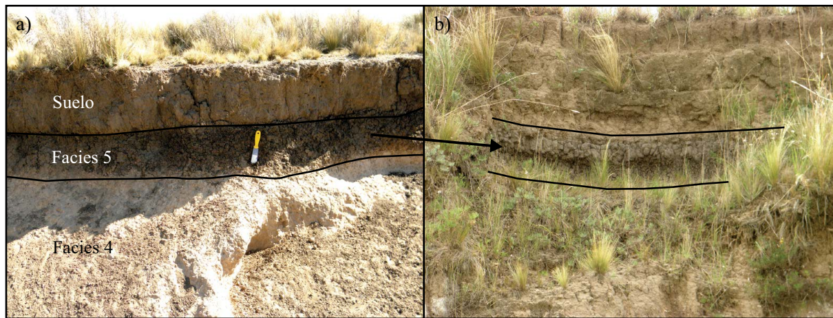
Figura 10. Arena limosa oscura maciza (facies 5). a) Contacto inferior (facies 4) y superior de esta facies en la localidad de Vaca Corral (escala= 22 cm); b) aspecto de esta facies en Pampa de Olaen, donde el desarrollo de prismas es mayor.
