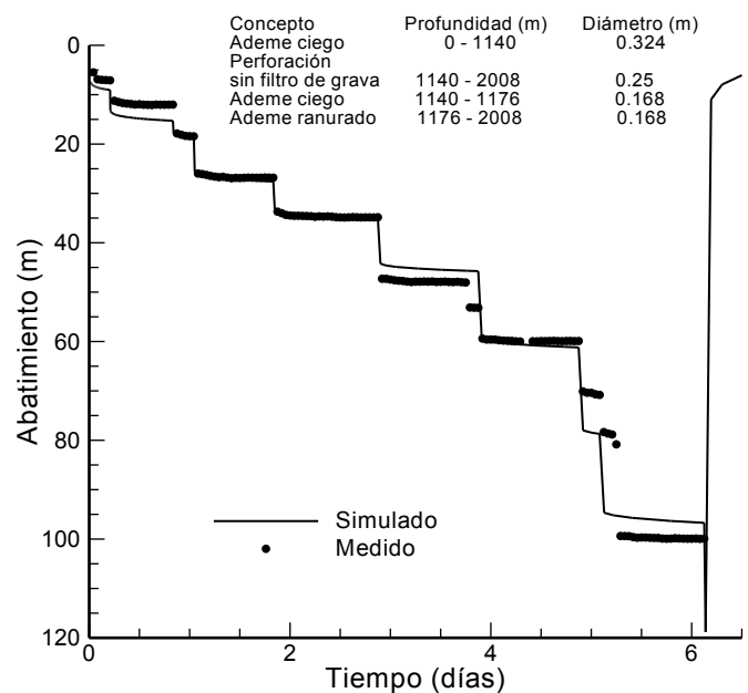
Figura 7. Simulación del aforo 3.
