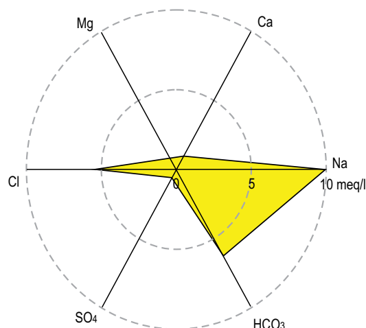
Figura 8. Diagrama radial de la composición de la muestra de agua M.
