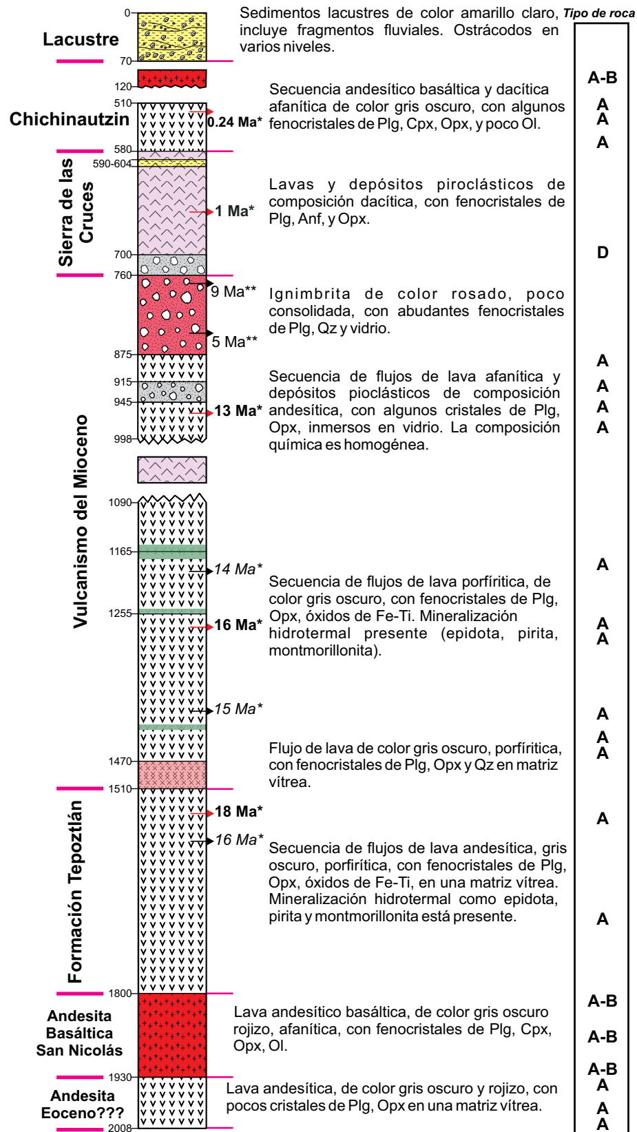
Figura 2. Corte litológico del pozo San Lorenzo Tezonco. Edades en millones de años (Ma) determinadas por los métodos de ^{40}\text{Ar}/^{39}\text{Ar} y ^{206}\text{Pb}/^{238}\text{U} en circones; las edades en negritas se consideran de mayor exactitud que aquellas en cursivas. Abreviaciones: A, andesita, D, dacita, A-B andesita basáltica (Modificado de Arce et al. , 2013).
