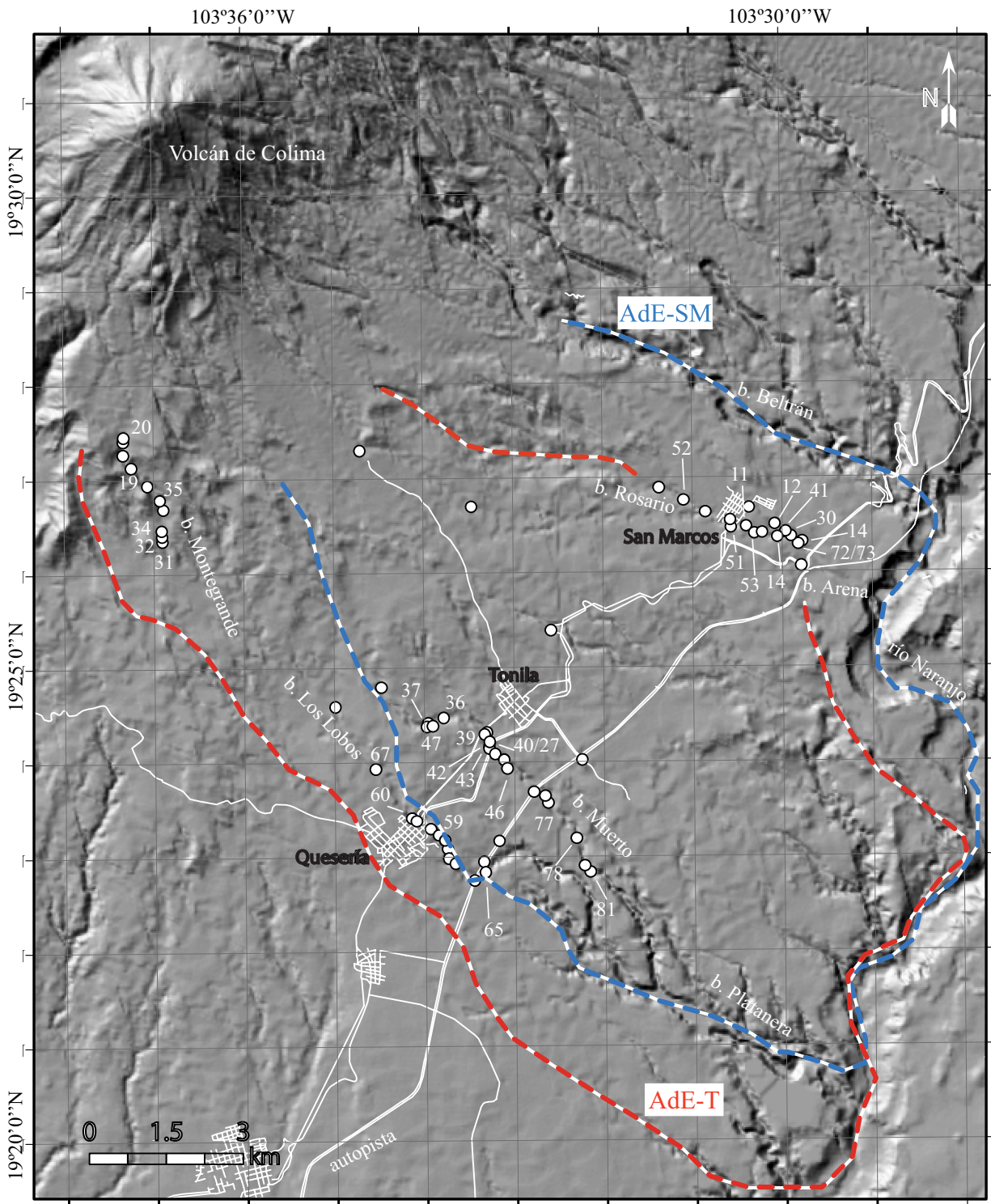
Figura 2. La imagen de elevación digital muestra la distribución de los depósitos de avalancha de escombros San Marcos (DAde-SM, línea discontinua azul) y Tonila (DAde-T, línea discontinua roja, así como los sitios investigados). Los puntos blancos indican los afloramientos con el número respectivo.
