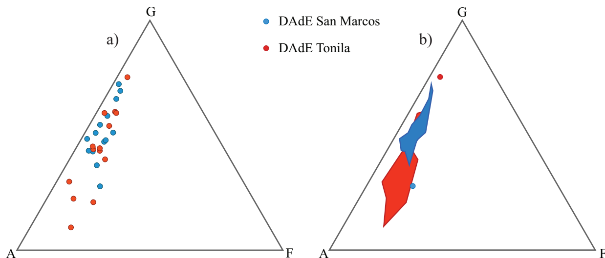
Figura 6. Diagramas triangulares Grava-Arena-Finos(Limo+Arcilla) de las muestras de los depósitos de avalancha de escombros (DAdE) San Marcos (a) y Tonila (b). El diagrama (a) representa los puntos gráficos de cada muestra recolectada, y el diagrama ternario (b) muestra las áreas de tendencia de los dos depósitos de avalancha de escombros.
