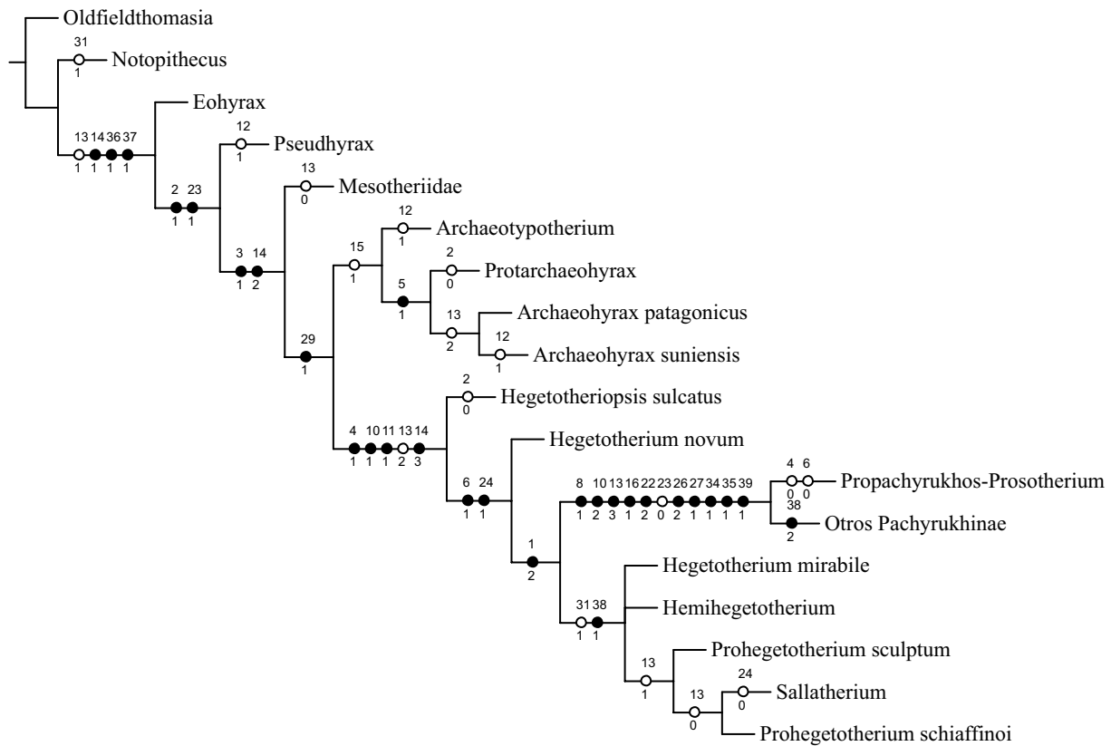
Figura 4. Único árbol más parsimonioso ( l=63 , ci=76 , ri=88 ) mostrando las relaciones filogenéticas de Hegetotheriopsis sulcatus n. gen. et sp., obtenido mediante búsqueda exhaustiva a partir de la matriz de datos morfológicos de Billet et al. (2009: apéndices 4 y 5) con la adición de los taxones discutidos en el texto (Tabla 2). Los estados de carácter indicados con círculos blancos indican homoplasias.
