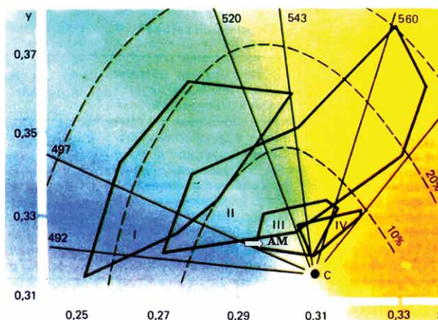
Figura 5. Gráfico colorimétrico de las amazonitas: pegmatitas de la Península de Kola (I) y de Urales (II); granitos de Transbaikal (III) y Kazajstán (IV). AM-amazonita mexicana. Modificada de Ostrooumov (1987).
