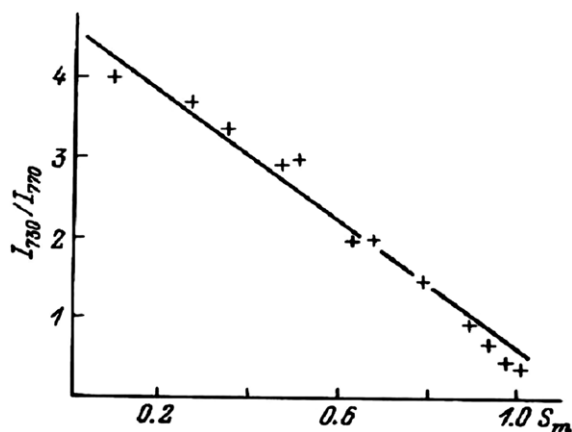
Figura 4. Correlación entre el valor espectrométrico ( I_{730}/I_{770} ) y el grado de desorden Al/Si estructural ( S_m ) en los feldespatos alcalinos: sanidina desordenada-microclina ordenada. Tomada de Ostrooumov (1991a).
