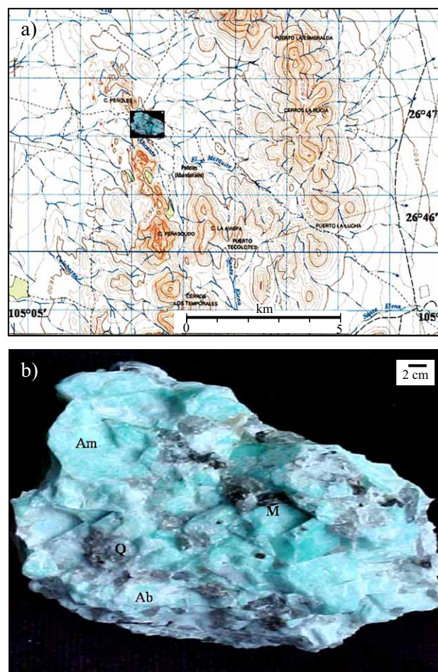
Figura 3. Localización del complejo granítico de composición subalcalina a) en el recorte de la carta topográfica (Pueblito de Allende, Chihuahua G13A59 esq. 1:50000, INEGI, 1994) y b) la amazonita azul en asociación con otros minerales principales componentes de la roca (Am-amazonita; Ab-albita; Q-cuarzo; M-mica. Cerros Bahues, Municipio Coronado).
