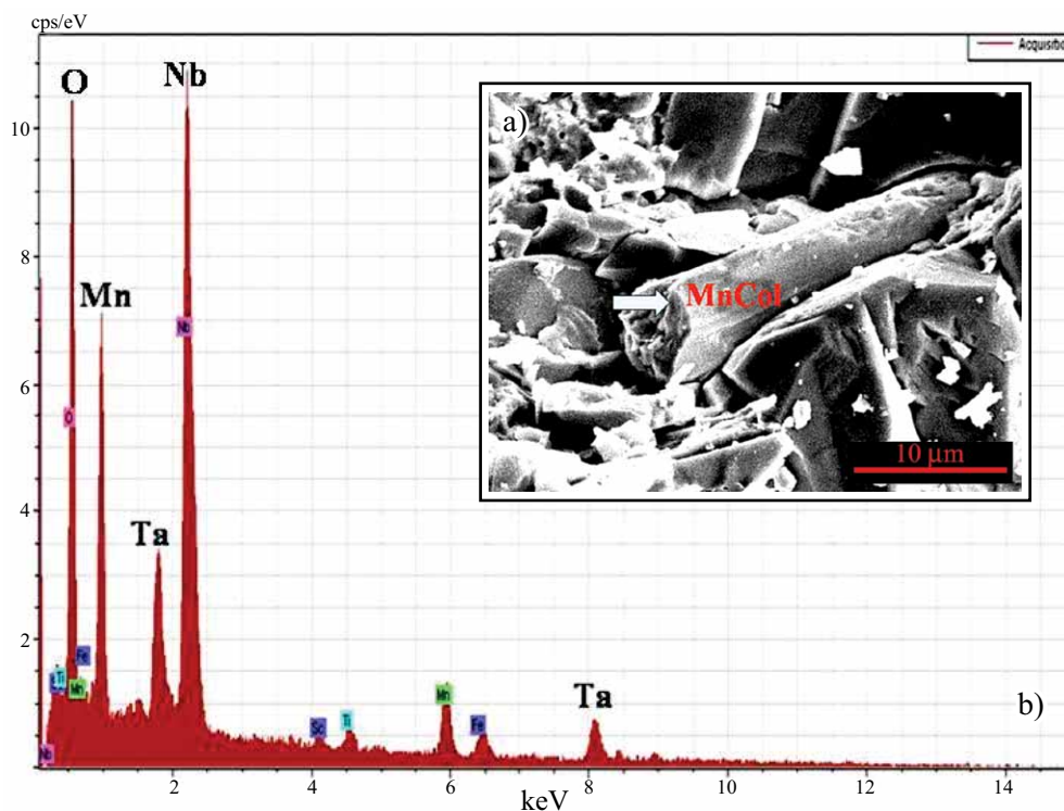
Figura 6. Fotomicrografía de MEB (a) y determinación de componentes (espectro EDS) (b) en un cristal de manganocolumbita (\text{Mn, Fe})(\text{Nb, Ta})_2\text{O}_6 procedente del yacimiento de amazonita de Cerros Bahues, Municipio Coronado, Chihuahua.
