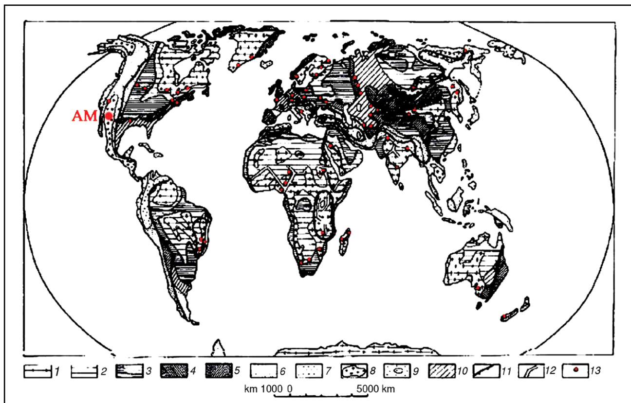
Figura 2. Distribución de los principales yacimientos de amazonita (esquema tectónico por Belousov, 1975): 1: escudos, 2: pendientes de escudos y anteclisas de plataformas antiguas, 3: sineclisas de plataformas antiguas, 4–7 : regiones de plegamiento (4: caledónicos, 5: hercínicos, 6: cretácicos (cimmeric), 7: alpinos), 8–9: macizos medianos en regiones de plegamiento, 10: plataformas epipaleozoicas con cubierta sedimentaria, 11: fronteras de cinturones neotectónicos y rifts, 12: grabens, 13: yacimientos de amazonita, 14–AM (amazonita mexicana). Modificada de Ostrooumov et al. (2008).
