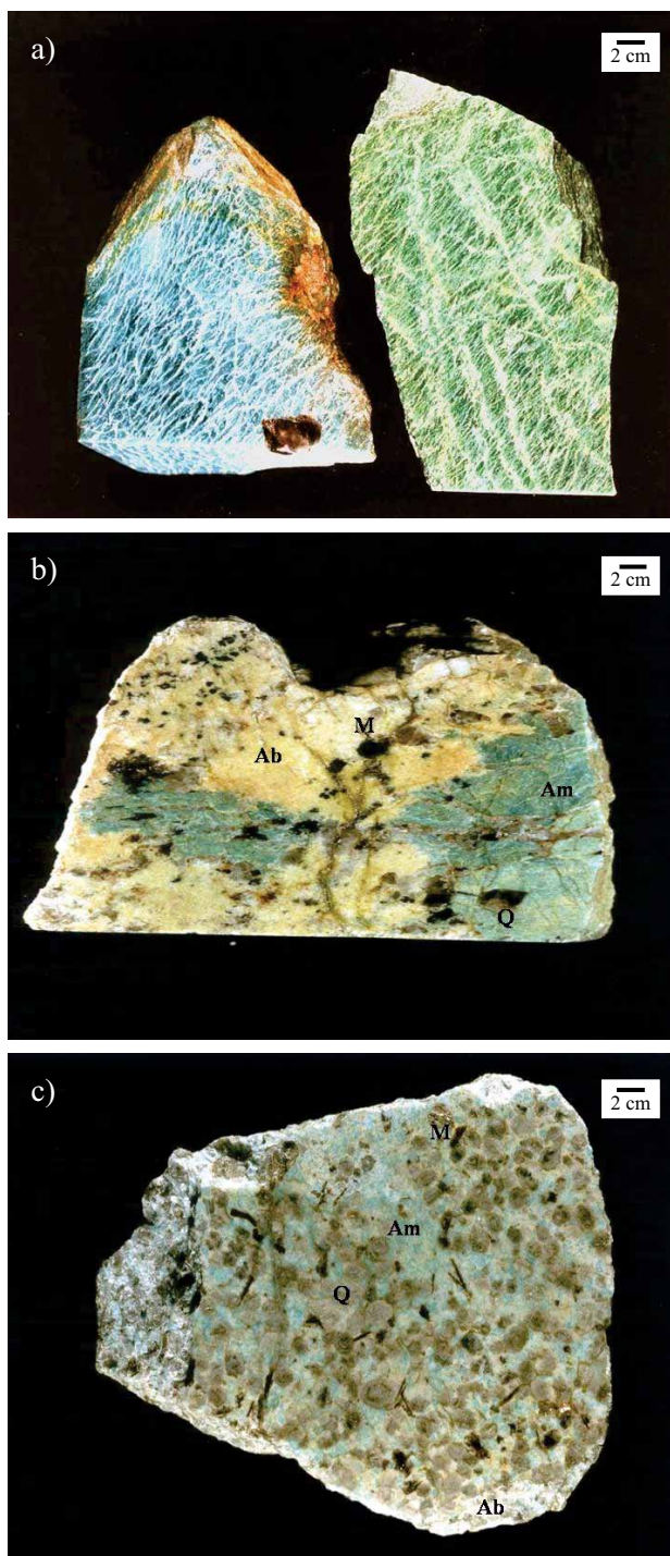
Figura 1. a-c. Gama de colores en diferentes ejemplares de amazonitas. Procedencias: a - pegmatitas precámbricas, b-pegmatitas paleozoicas, c- granitoides mesozoicos (Am-amazonita; Ab-albita; Q-cuarzo; M-mica).
