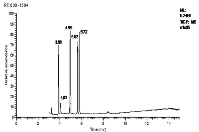
Figura 2. Cromatograma con los picos correspondientes a: \alpha -pinoeno (tiempo de retención, R_t = 3.47 ), \alpha -tujeno ( R_t = 3.88 ), 6,6-dimetil-2-metilenbicyclo[3,1,1]heptano ( R_t = 4.03 ), (E)-10 tagetona ( R_t = 4.95 ), verbenona ( R_t = 5.63 ) y crisantenona ( R_t = 5.72 ).
