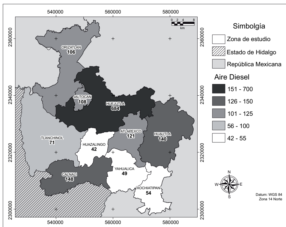
Fig. 3. Distribución por municipio de las emisiones de contaminación atmosférica por fuentes móviles en base a diesel (ton/año)
