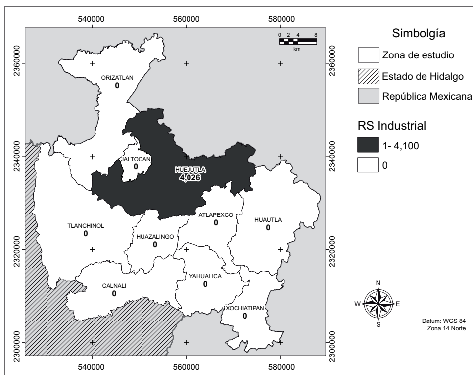
Fig. 6. Distribución por municipio de las emisiones de contaminación al suelo por fuentes industriales (ton/año)
