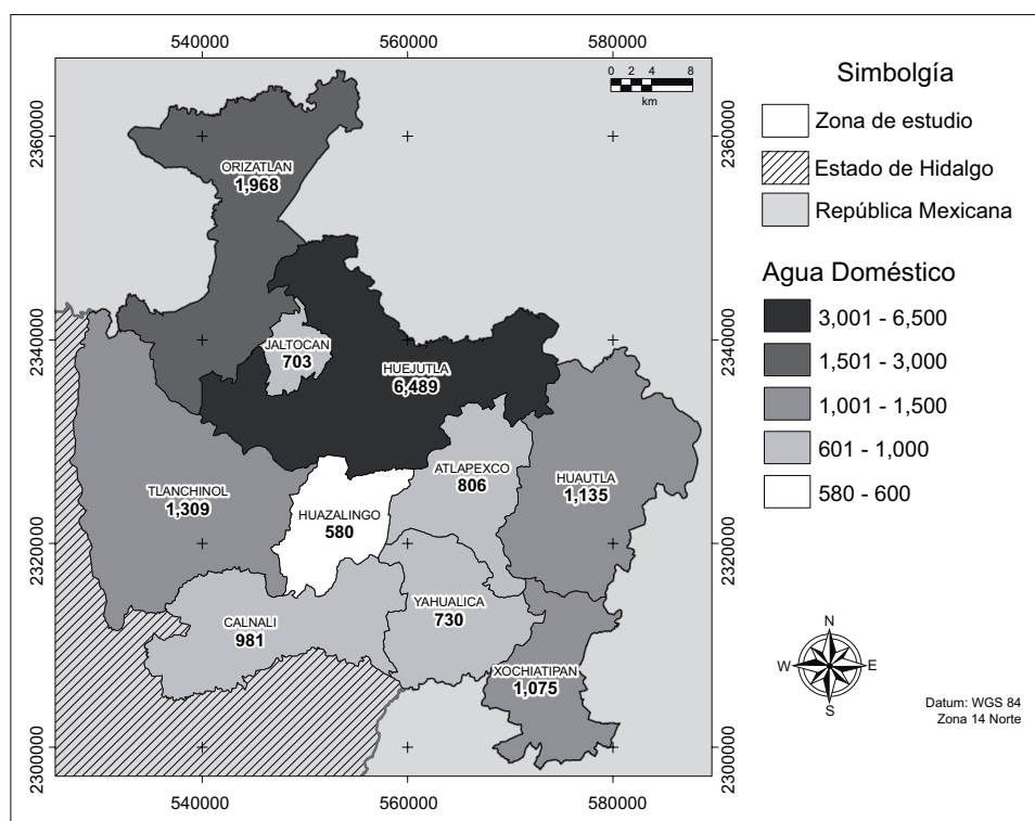
Fig. 5. Distribución por municipio de las emisiones de contaminación al agua por fuentes domésticas (ton/año)
