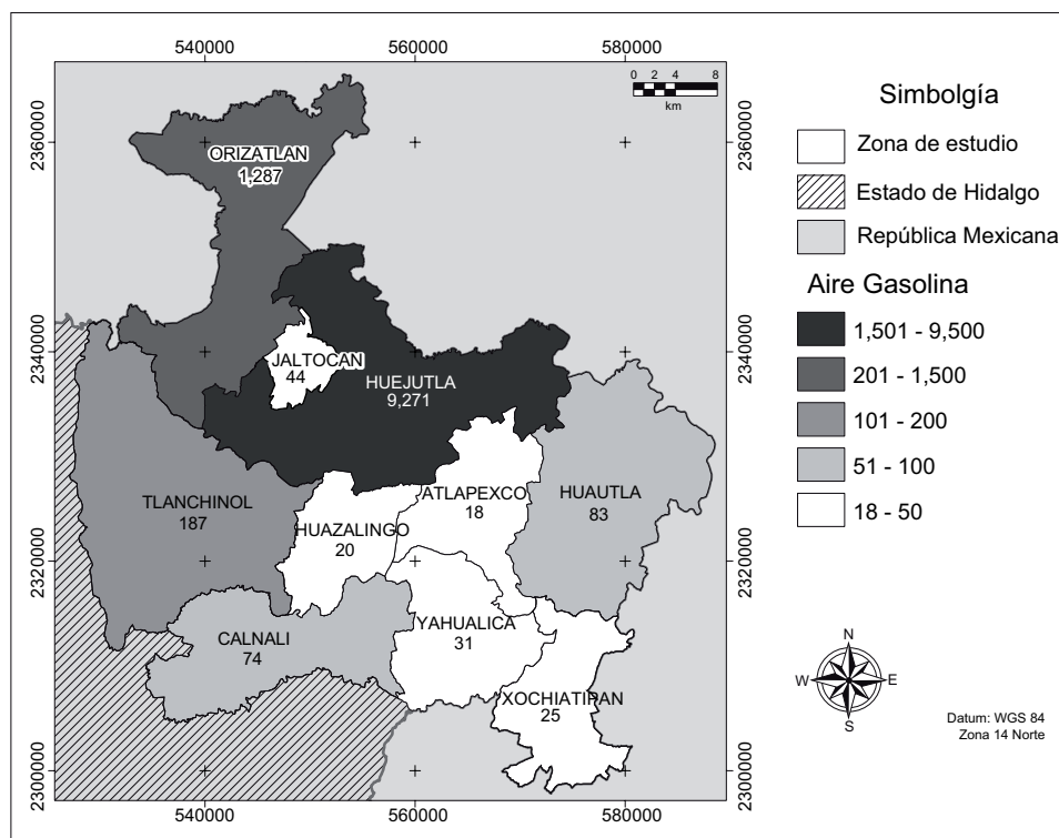
Fig. 2. Distribución por municipio de las emisiones de contaminación atmosférica por fuentes móviles en base a gasolina (ton/año)
