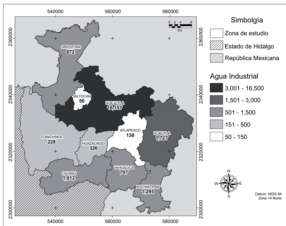
Fig. 4. Distribución por municipio de las emisiones de contaminación al agua por fuentes industriales (ton/año)
