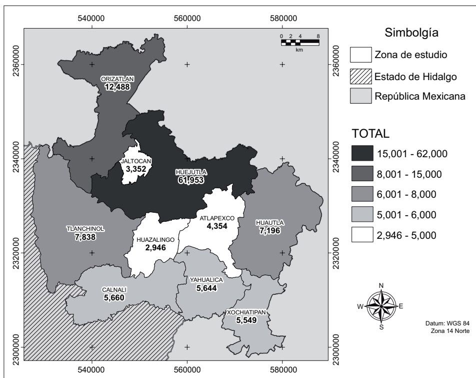
Fig. 8. Distribución por municipio de las emisiones de contaminación en aire, agua y suelo en la región de la Huasteca Hidalguense (ton/año)
