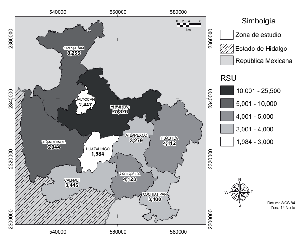
Fig. 7. Distribución por municipio de las emisiones de contaminación al suelo por RSU (ton/año)
