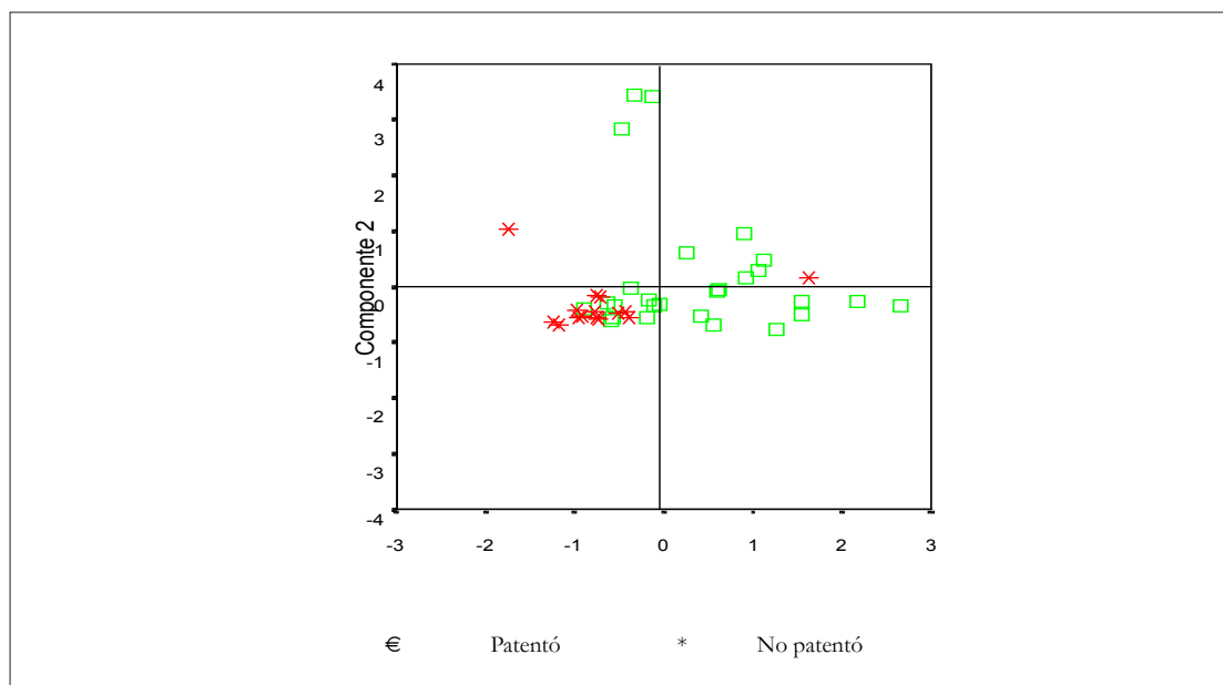
Gráfico 1 Componentes en espacio rotado
