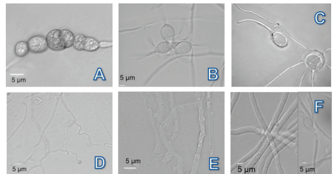
Figura 3. Microfotografías de hongos nematófagos aislados de suelo de zonas productoras de chile Bell Pepper en el Valle del Fuerte, Sinaloa. A - C) Clamidosporas, conidios y anillos no constrictores de Dactylella ; D y E) Nódulos y micelio adhesivo de Nematoctonus e incisivo; y F) Red de hifas y conidio de Arthrobotrys .
