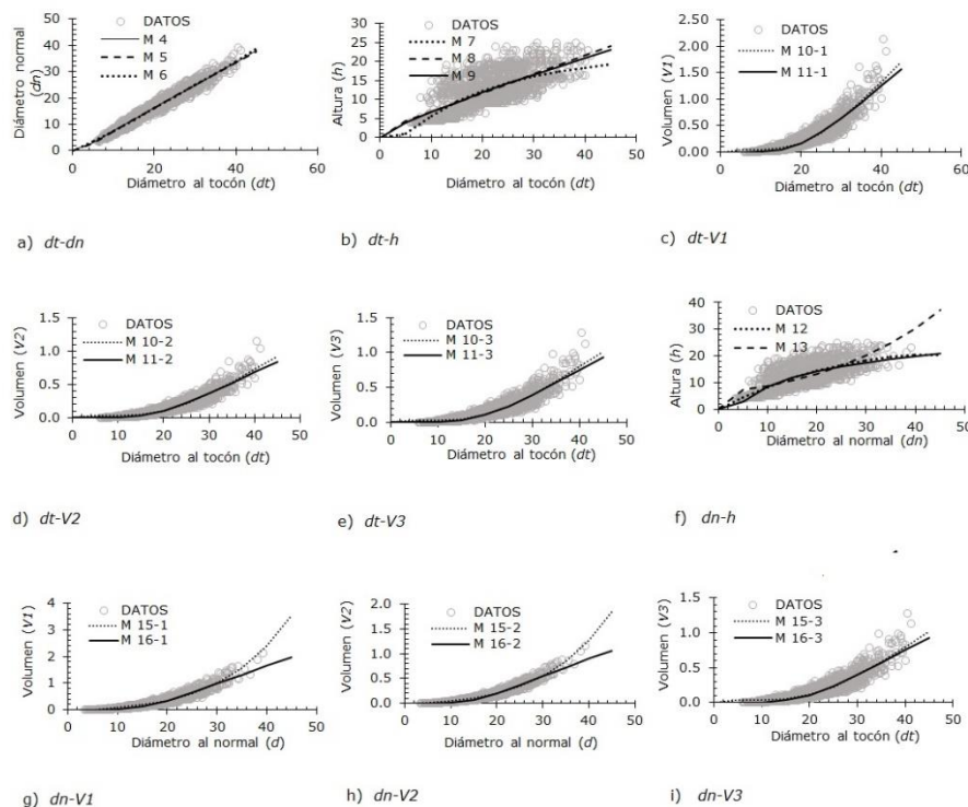
Figura 2. Predicción de las relaciones alométricas versus datos observados en diámetro de tocón ( dt ), diámetro normal ( d ), altura total ( h ) y volumen ( V ) para plantaciones forestales de Pinus patula Schiede ex Schltdl. et Cham. en el Estado de México.
