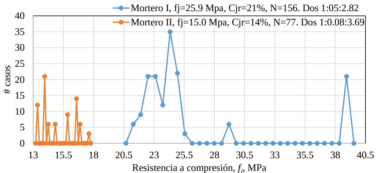
Figura 8. Polígonos de frecuencias de la resistencia a compresión en morteros I y II
