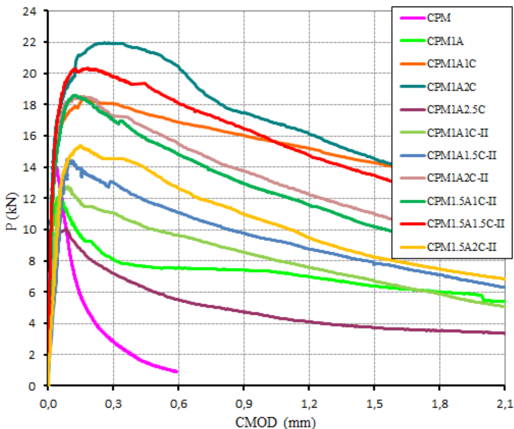
Figura 6. Curvas P-CMOD dos compósitos de microconcreto
