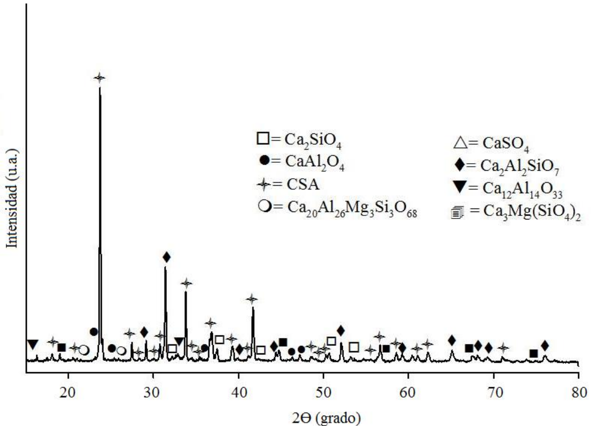
Figura 1. Patrón de DRX del sintetizado a 1250 °C.
