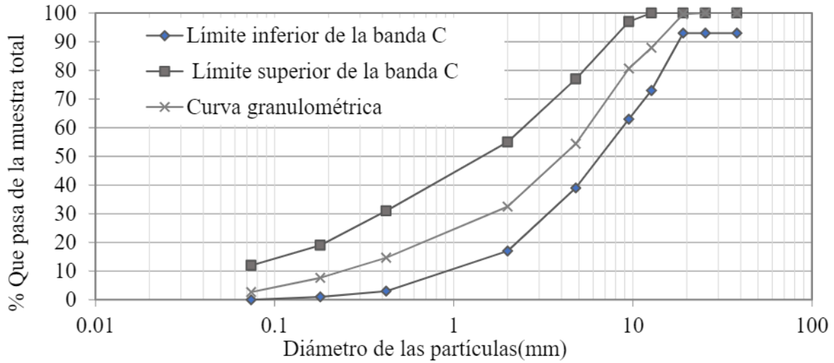
Figura 1. Curva granulométrica de las mezclas.
