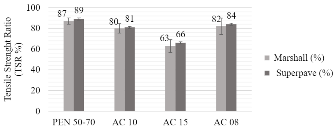
Figura 5. Resultados del ensayo de daño por humedad inducida para cada mezcla.
