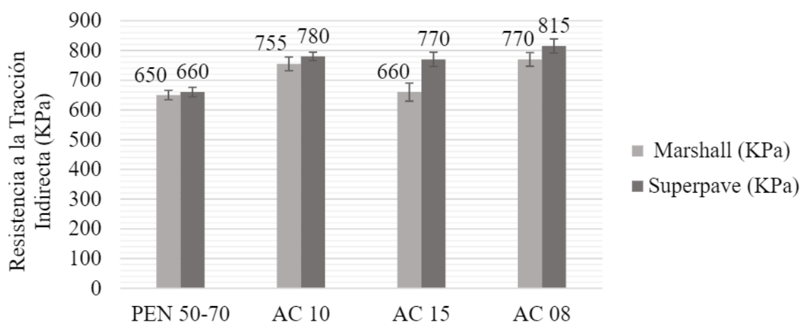
Figura 3. Resultados del ensayo de RT para cada mezcla.
