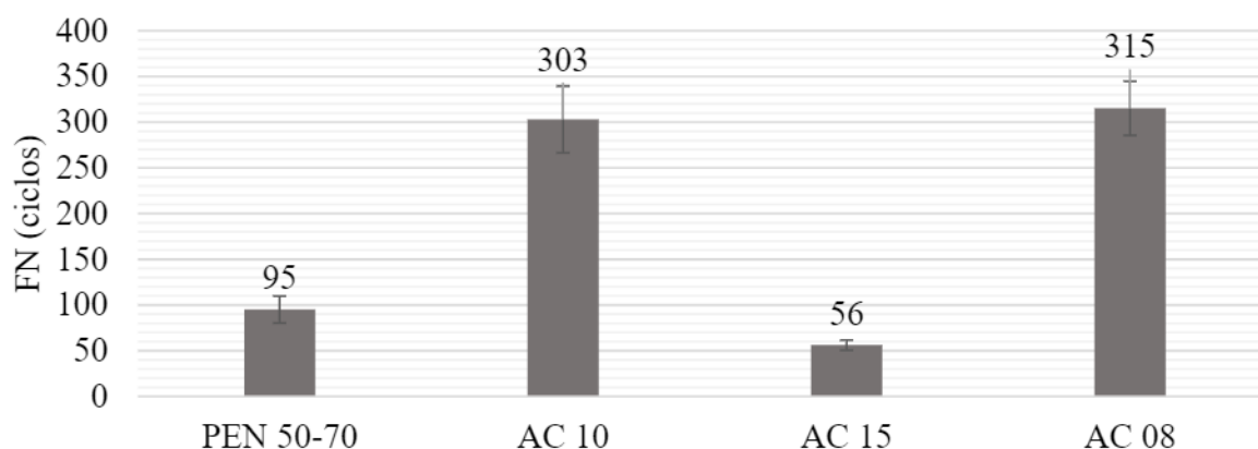
Figura 6. Resultados del ensayo de FN.
