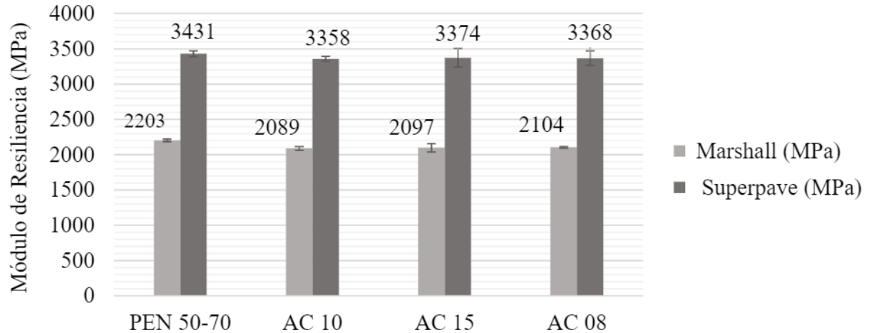
Figura 4. Resultados del ensayo de MR para cada mezcla.
