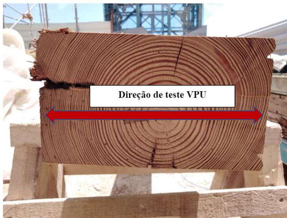
Figura 10. Esquema de aplicação VPU perpendicular à fibra
