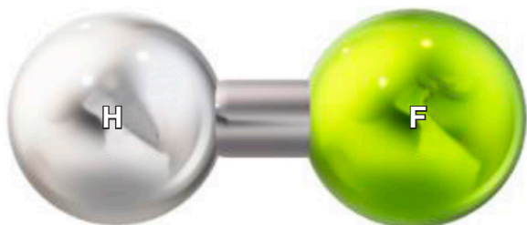
Figura 1: Estructura tridimensional del fluoruro de hidrógeno.
