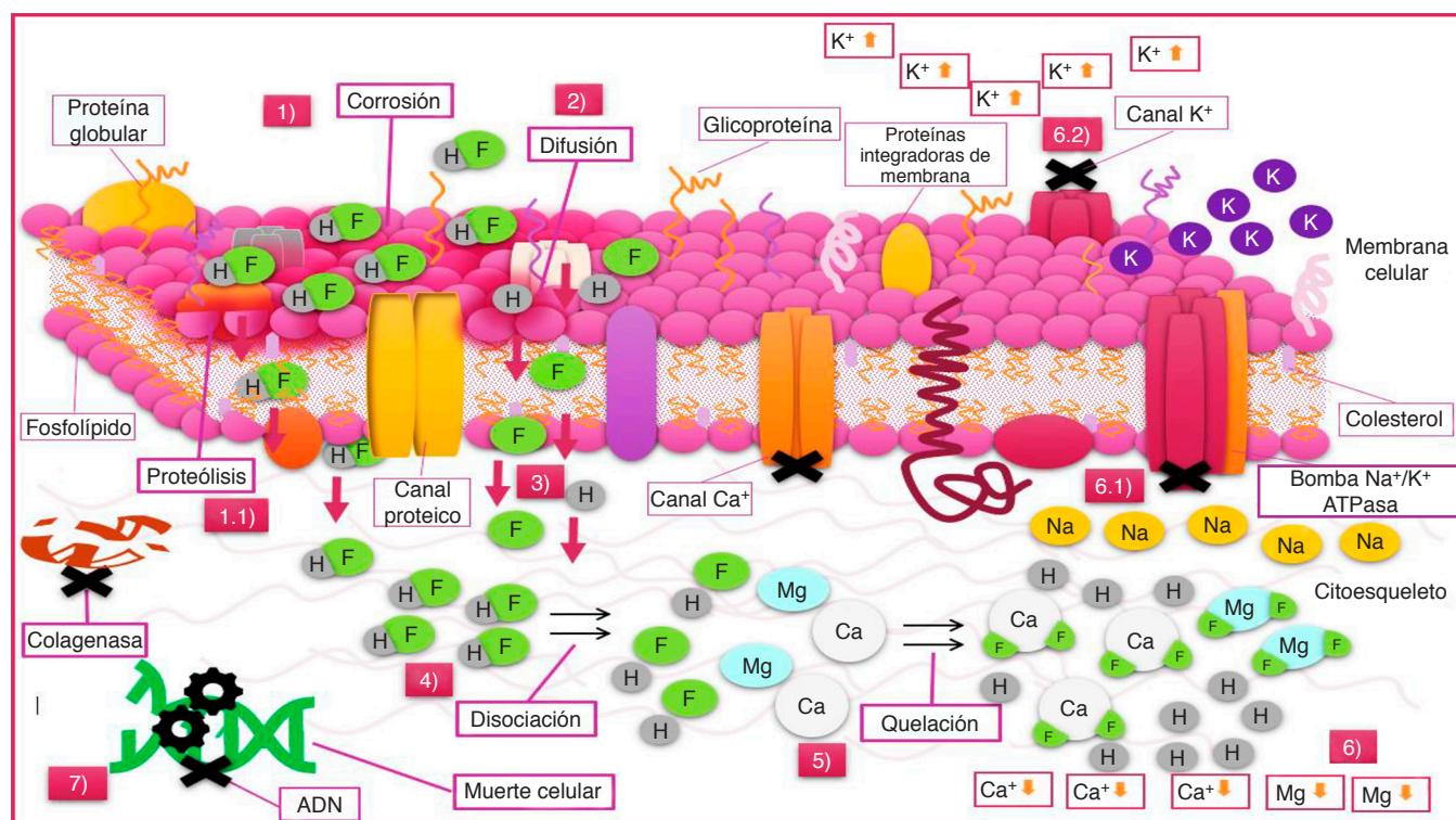
Figura 3: Mecanismo de lesión intracelular del ácido fluorhídrico. Al entrar en contacto con la membrana celular se inicia un proceso químico corrosivo (1), el cual genera proteólisis modificando la estructura celular (1.1), por mecanismo de difusión (2) en forma compuesta y disociada, penetra a través de la membrana hasta el espacio intracelular (3), continúa disociándose (4) resultando en iones de hidrógeno y fluoruro, los cuales por quelación (5) forman compuestos insolubles en contacto con iones de calcio y magnesio, disminuyendo su concentración intracelular (6), lo que conlleva a bloqueo de canales de calcio, inactivación de la bomba sodio-potasio ATPasa (6.1) que impiden el paso de potasio al interior de la célula, aumentando su concentración extracelular (6.2). Como consecuencia de lesión directa a nivel de la membrana y del intercambio iónico, se inhiben mecanismos de reparación por acción de las colagenasas y a nivel del ADN (7), condicionando muerte celular.
