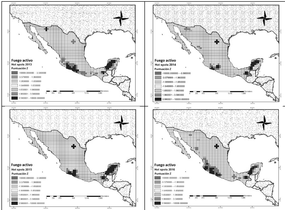
Ilustración 2. Agrupación de ocurrencia de incendios 2005-2016. Norte, Occidente y Península de Yucatán.
