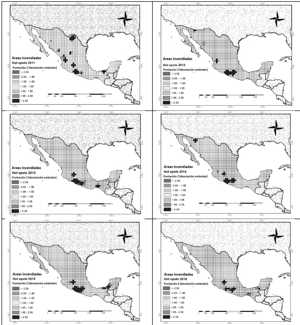
Ilustración 1. Agrupación de áreas incendiadas 2005-2016. Norte y Occidente de México.
