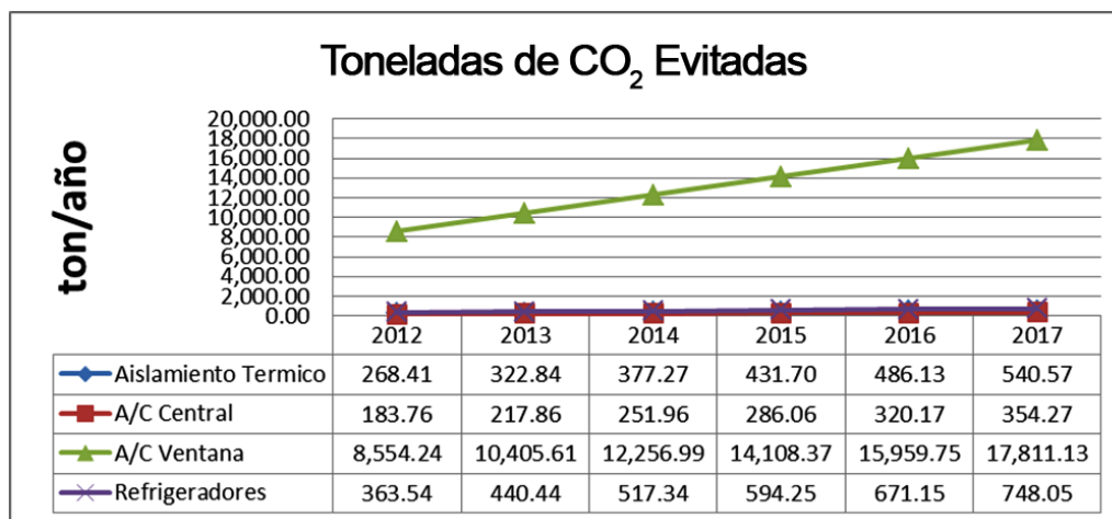
Figura 5. Prospectiva de las emisiones de CO 2 evitadas hasta el año 2017.
