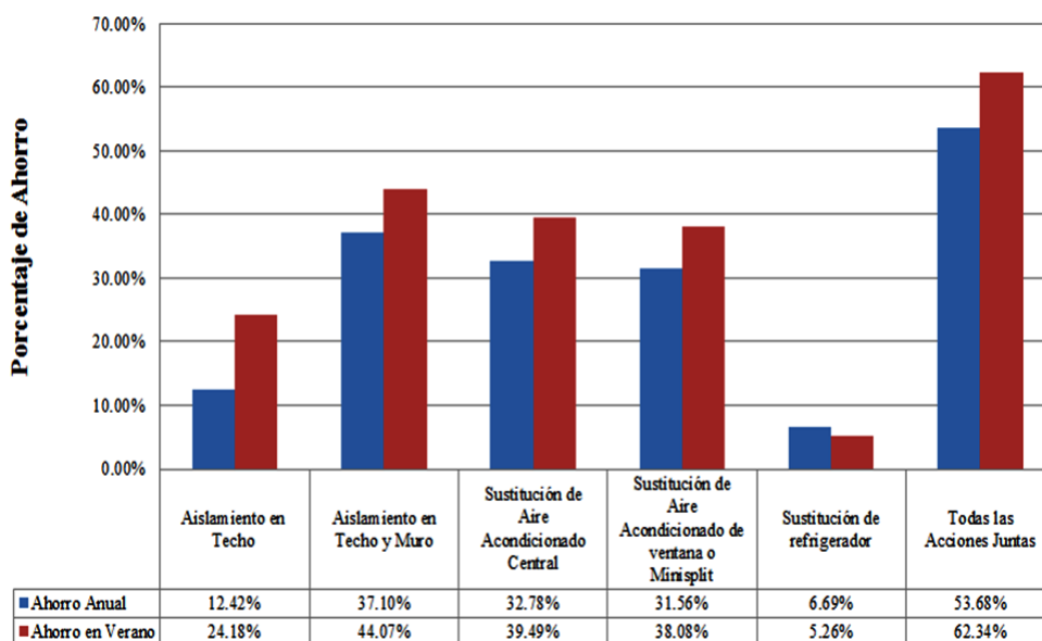
Figura 3. Porcentajes de ahorro de energía eléctrica para cada subprograma del programa ASI.
