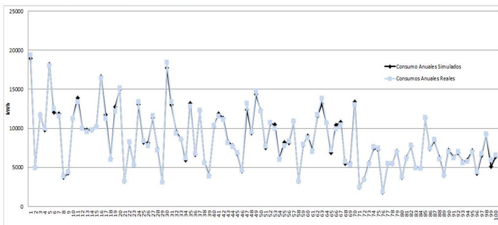
Figura 1. Comparativo anual de los consumos eléctricos simulados contra los registrados en el recibo eléctrico de las viviendas encuestadas.
