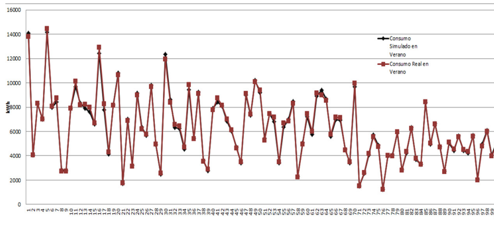
Figura 2. Comparativo para los meses de verano de los consumos eléctricos simulados contra los registrados en el recibo eléctrico de las viviendas encuestadas.
