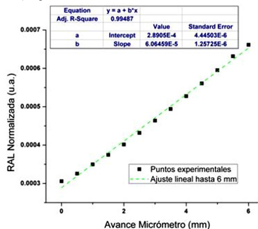
Figura 12. Grafica de señal RAL normalizada vs. Incremento de flexión (flecha), rango hasta 6 mm.
