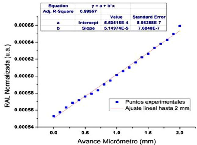
Figura 10. Grafica de señal RAL normalizada vs. Incremento de flexión (flecha), rango hasta 2 mm.
