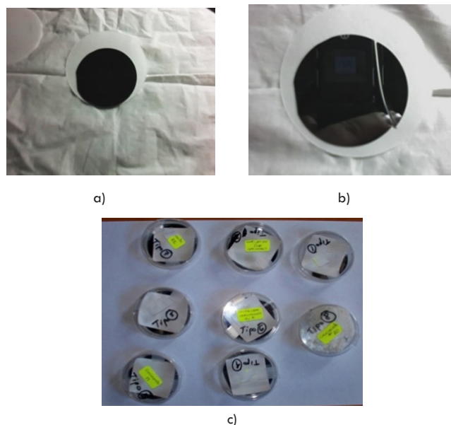
Figura 5. Cristales Derivados, se clasifican y registra su posición original en la oblea. a) Oblea entera de Si (110), b) Corte inicial del cristal de Si, c) Cristales clasificados.
