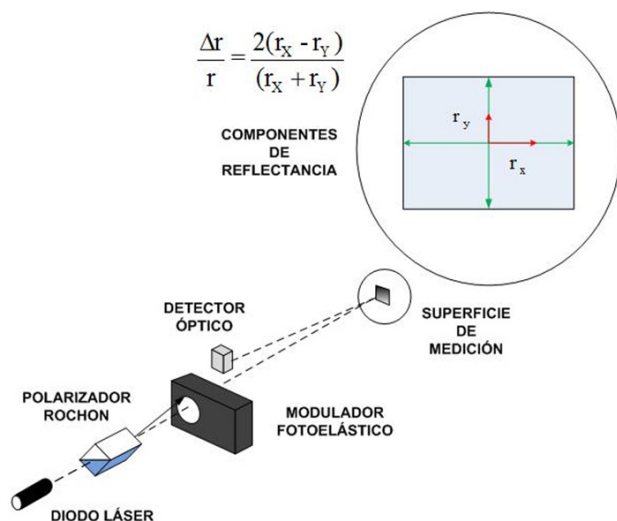
Figura 2. Sistema RAL, rayo incidente ortogonal a la optogalga, y detalle de las componentes de reflectancia.
