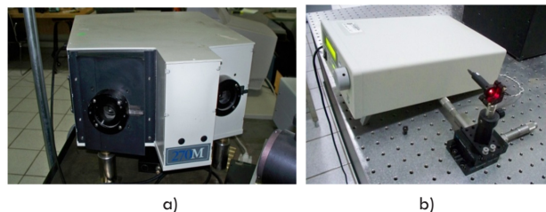
Figura 3. a) Monocromador utilizado para RAS. b) Diodo láser con fuente utilizado para RAL.
