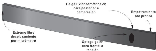
Figura 9. a) Visualización de deformación de viga instrumentada en Flexor Vishay™, puntos de colocación de optogalga y galga extensométrica.
