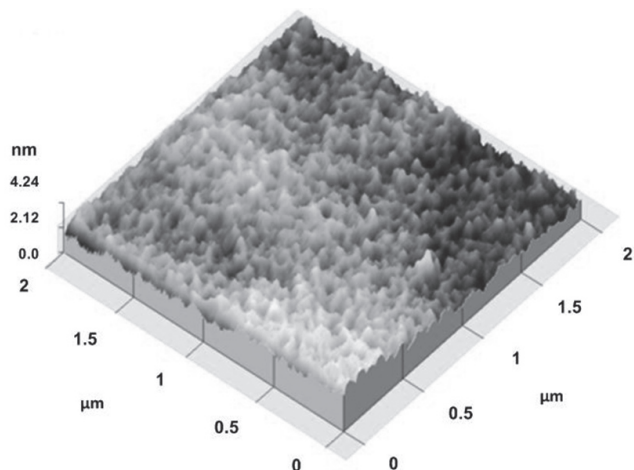
Figura. 7. Imagen por microscopía de fuerza atómica (AFM) de la superficie de la optogalga, presenta baja rugosidad (2.12 a 4.24 nm), esta superficie con acabado tipo espejo presenta gran reflectividad especular y bajo esparcimiento de luz.
