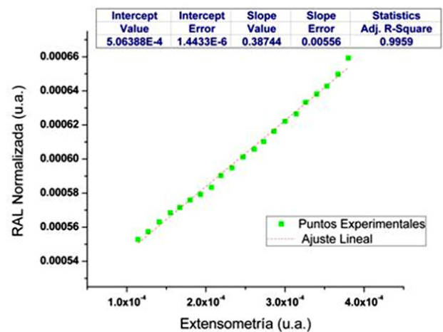
Figura 11. Grafica de RAL normalizada vs. Señal de Extensometría. Rango hasta 2 mm.
