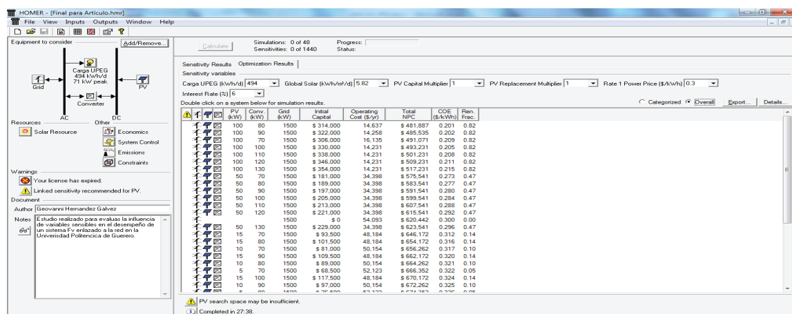
Figura 4. Resultados de la simulación y optimización del sistema estudiado para 0.3 $/kWh (PV es la capacidad del sistema fotovoltaico; Conv. es la capacidad del convertidor; Grid es la capacidad de la red eléctrica; Initial Capital es la inversión inicial; Operating Cost es el costo de operación anual; Total NPC es el costo presente neto total; COE es el costo de la energía y Ren. Frac. es la fracción de energía que es suministrada por las tecnologías renovables)
