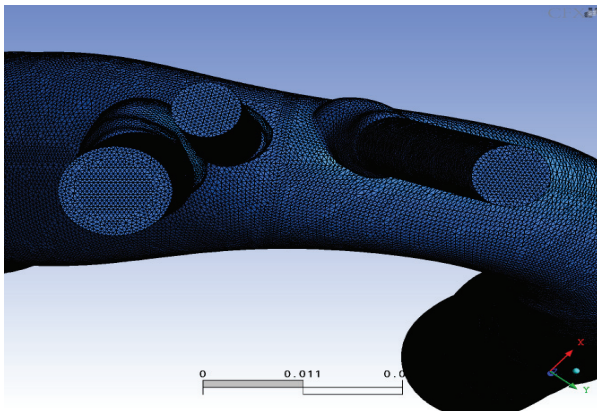
Figura 6. Detalle de la malla de cálculo. Vista superior (céfalo-caudal) desde la perspectiva de plano transversal superior al dominio. De izquierda a derecha se observan el tronco braquicefálico, la carótida izquierda y la subclavia izquierda
