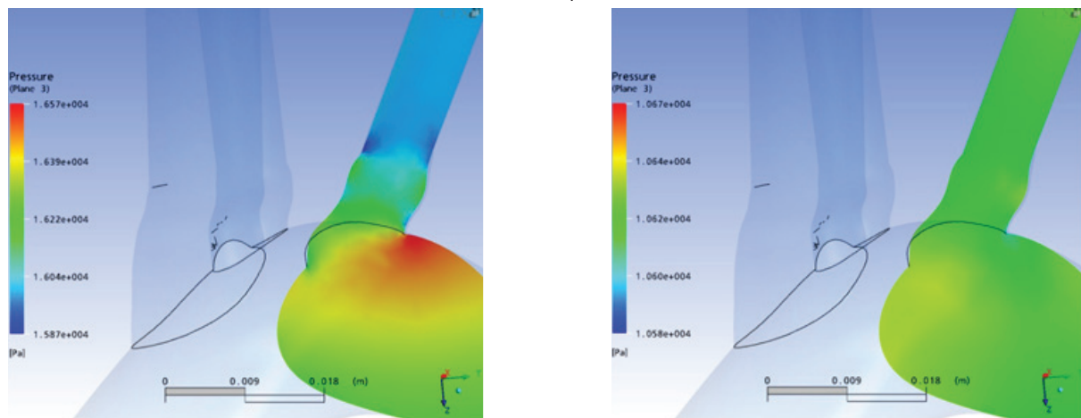
Figura 12. Detalle de la distribución de presiones a los 90° y 270° del ciclo cardíaco en la raíz de las tres ramas del cayado aórtico
