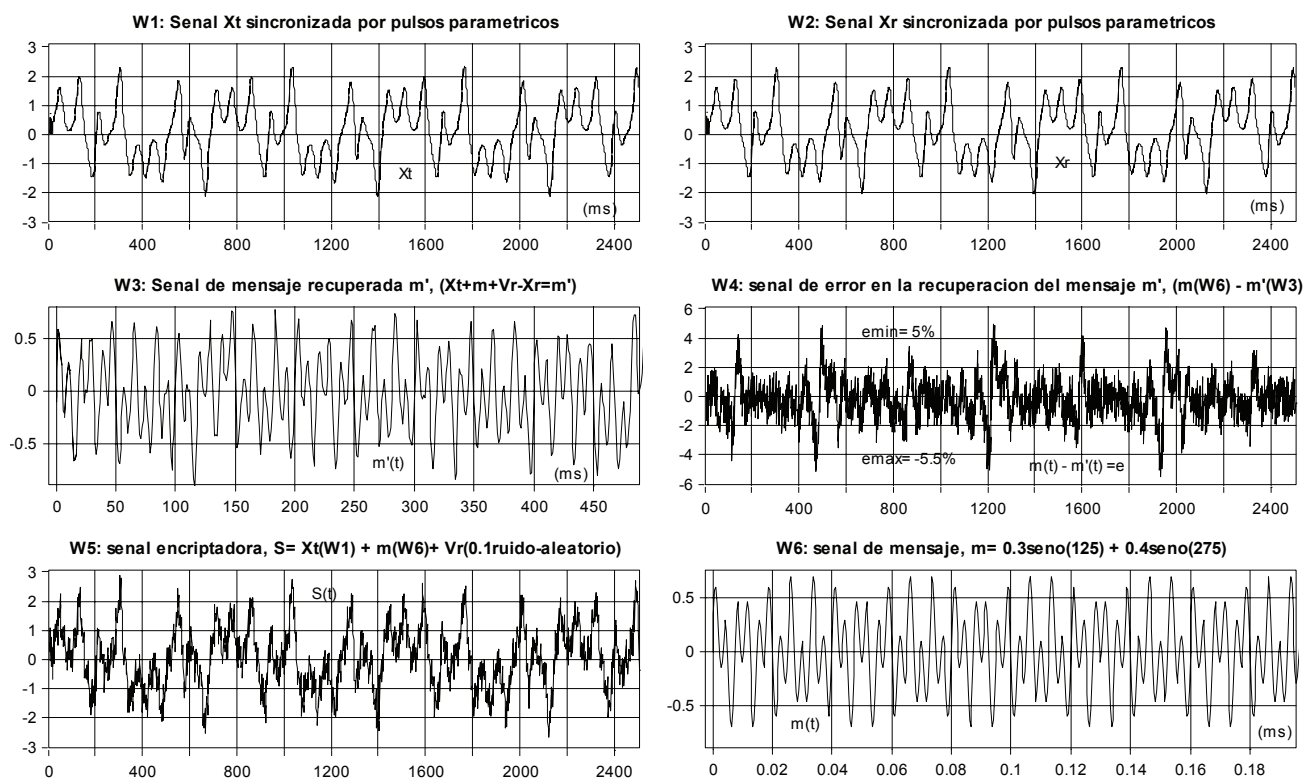
Figura 11. La sincronización atípica en una aplicación de encriptamiento por suma descrita en el programa Dadisp. La ventana W4 presenta un error del 5.5% en la recuperación del mensaje original
