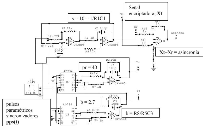
Figura 3. Circuito de Lorenz (receptor) mostrando sus parámetros y variables descriptivas. Se indica la señal de asincronía como calificadora de la sincronización entre los circuitos en atención a los pps(t)
