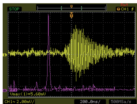
(b) Cavidad \varnothing = 2 mm en aislamiento - cable MT
