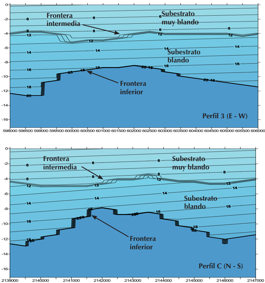
Figura 8. Perfiles 3 y C que muestran la variación espacial de la resistencia al corte
