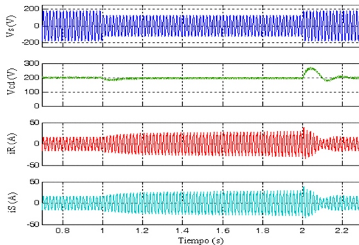
Figura 8. Estado transitorio cuando ocurre un sag de voltaje
