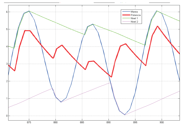
Figura 4. Generación con un embalse en modo de reflujo y generación con doble embalse (azul marea, verde nivel en el embalse, rojo potencia)
