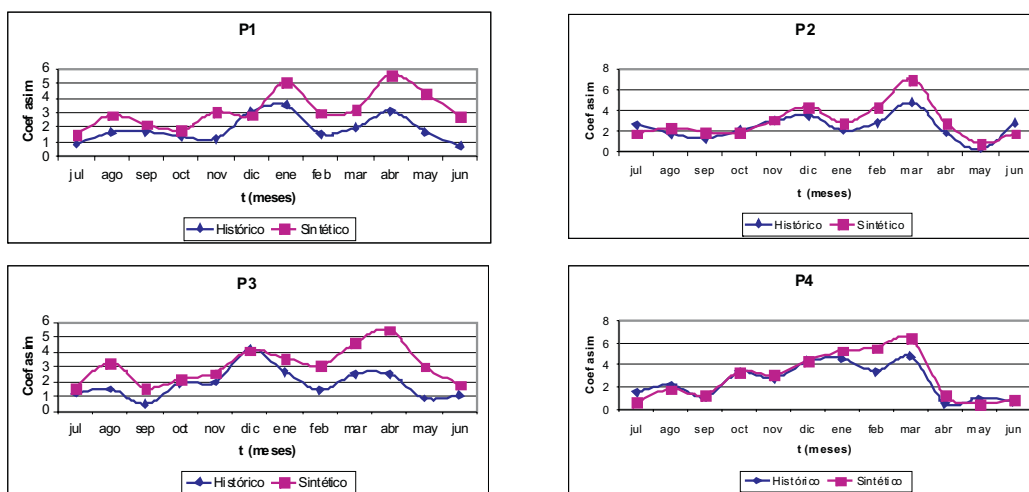
Figura 8. Comparación de los coeficientes de asimetría
