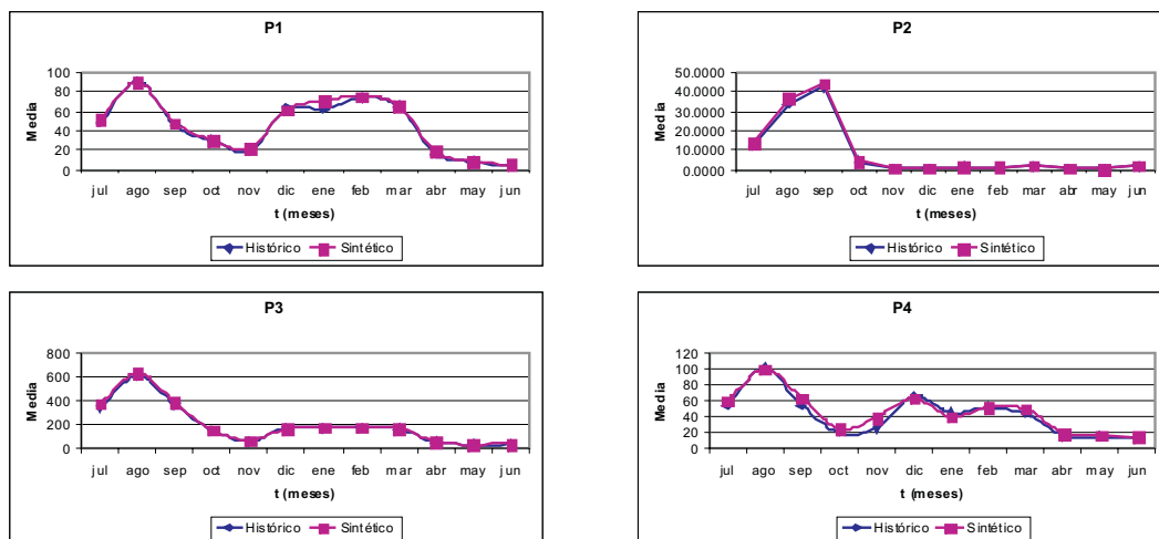
Figura 6. Comparación de las medias ( hm^3 )
