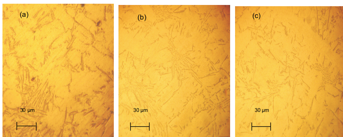
Figura 4. Fotomicrografías de las muestras A5 (a), A15 (b) y A25 (c)
