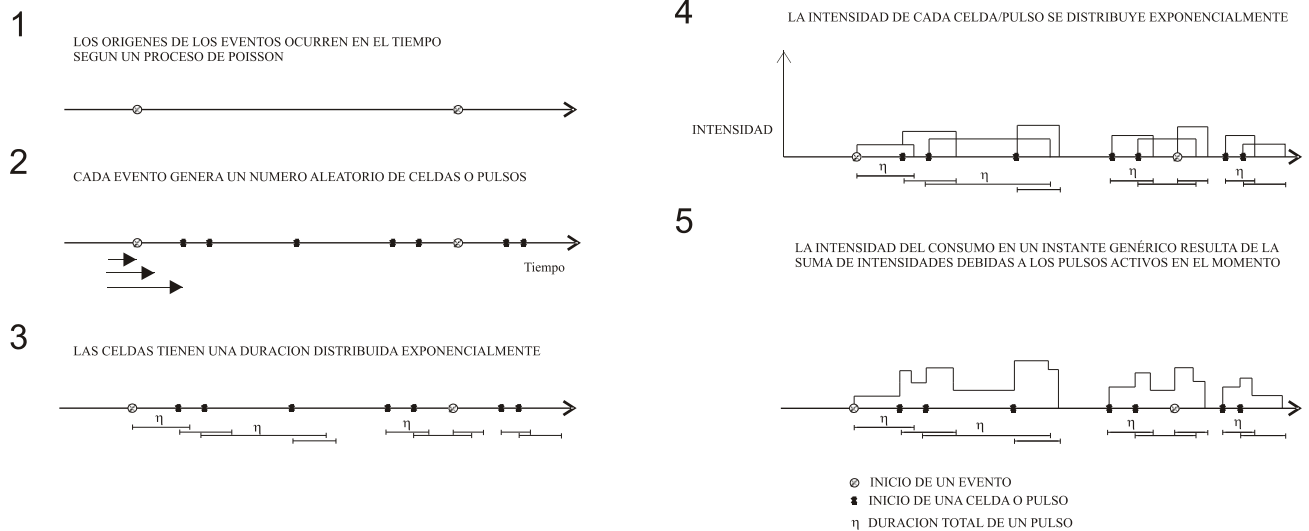
Figura 1. Esquemización del modelo Neyman-Scott, (Cowpertwait, 1991)
