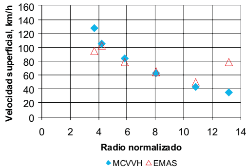
(a) Huracán Isidoro ( B=1.20 )
