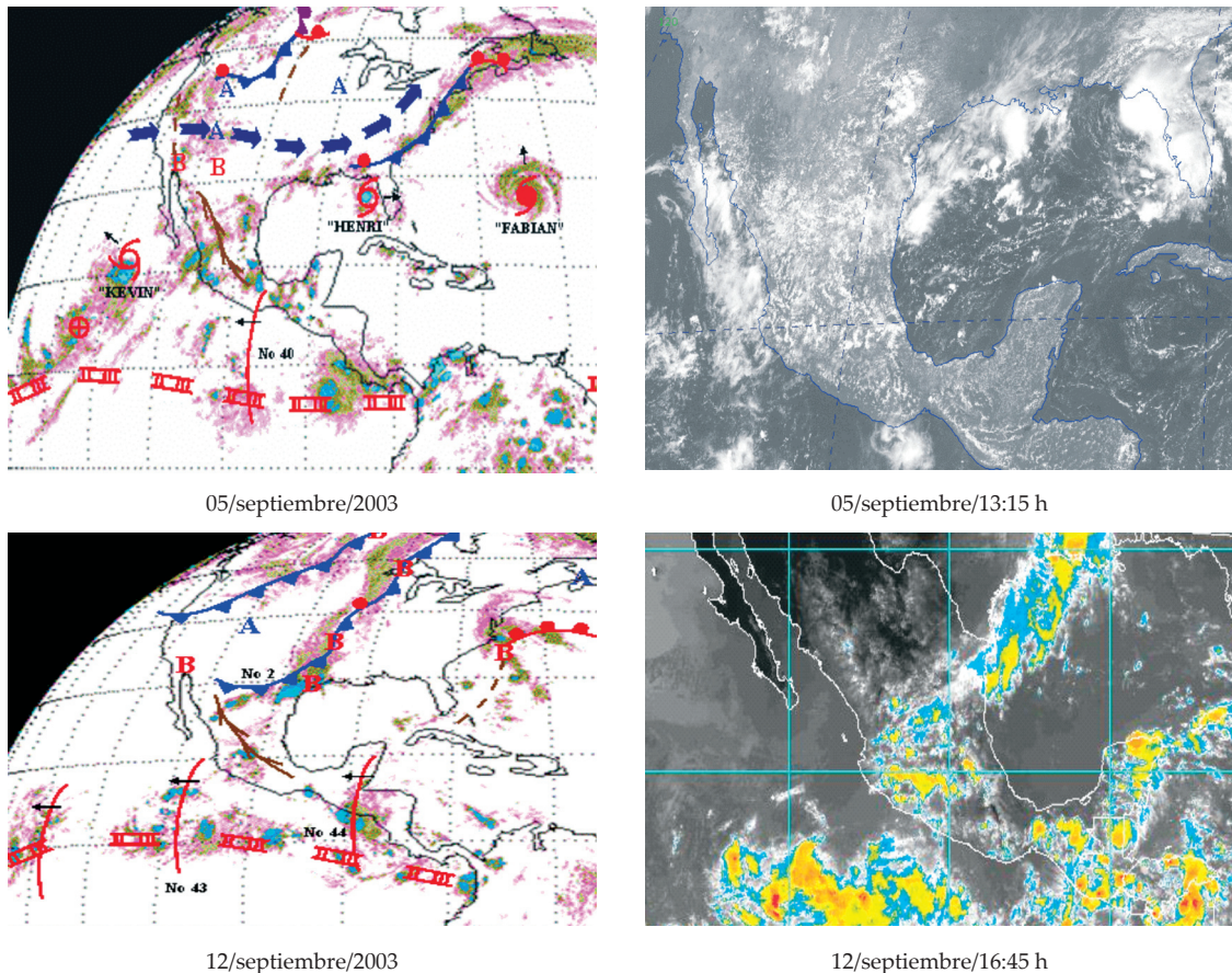
Figura 3. Fenómenos meteorológicos e imágenes de satélite de septiembre de 2003, donde se observan las bandas nubosas sobre el centro del país causantes de las lluvias intensas en el estado de Guanajuato.
