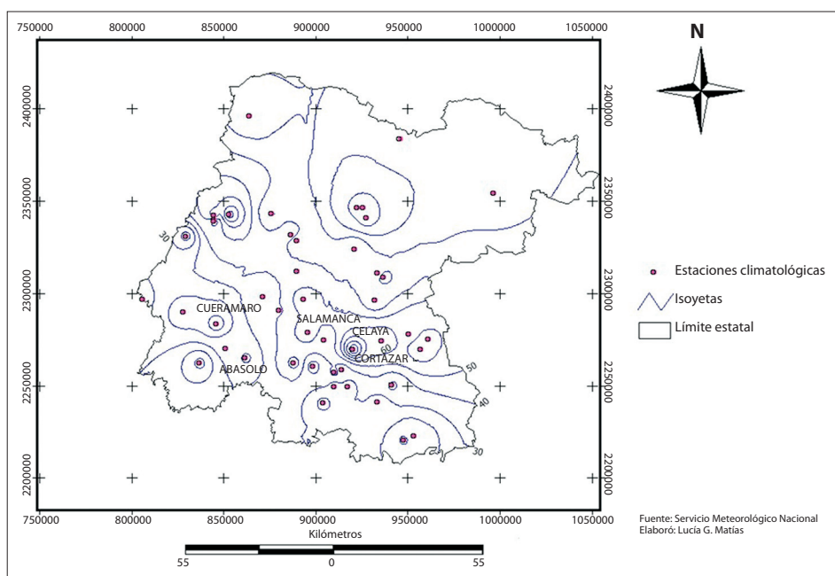
Figura 4a. Isoyetas del 6 de septiembre de 2003. El núcleo máximo se localiza al sureste de Celaya con un valor mayor de 90 mm en la estación Cortazar.
