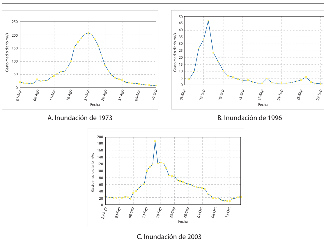
Figura 7. Hidrogramas de la estación Las Adjuntas para diferentes inundaciones.
