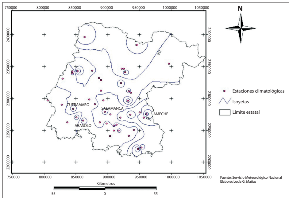
Figura 4b. Isoyetas del 4 al 18 de septiembre de 2003. El valor máximo fue reportado en la estación Amealco con más de 300 mm.
