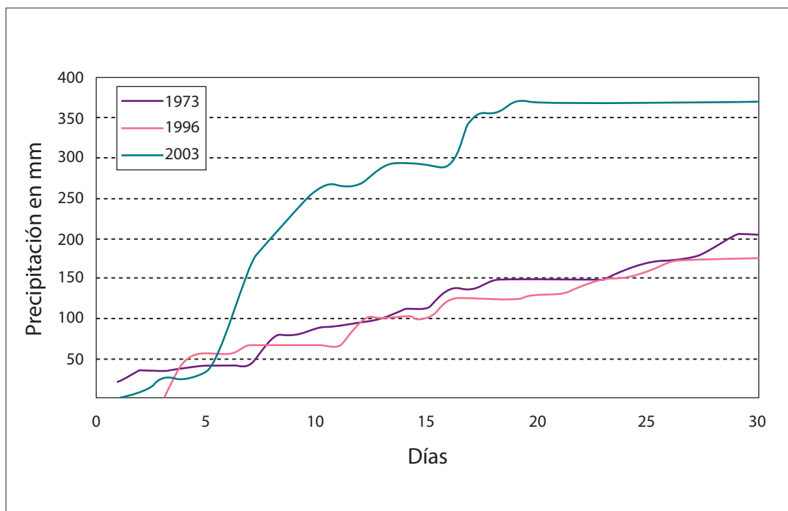
Figura 6. Precipitación acumulada de las inundaciones de 1973, 1996 y 2003.
