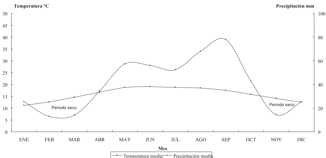
Figura 2. Definición de periodos secos en el ejido Corona del Rosal.
