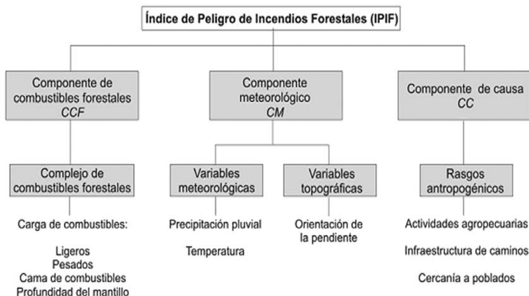
Figura 3. Modelo conceptual propuesto para la evaluación del peligro de incendios forestales.
