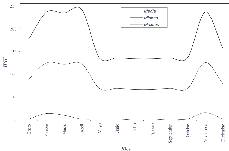
Figura 10. Distribución temporal de los valores estandarizados mínimos, máximos y promedio del Índice de Peligro de Incendios Forestales.
