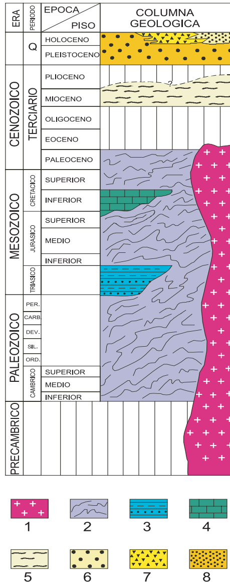
Figura 3. Columna geológica del área estudiada. Tipos litológicos: 1. Granitos, granodioritas; 2. Gneises cuarzo-feldespáticos, esquistos de biotita; 3. Areniscas, limonitas, conglomerados, pizarras, filitas y esquistos; 4. Calizas; 5. Derrames lávicos con depósitos piroclásticos y horizontes tobáceos; 6. Depósitos litorales, arenas; 7. Depósitos detríticos, coluvio-proluviales; 8. Depósitos aluviales, arenas, arcillas.
