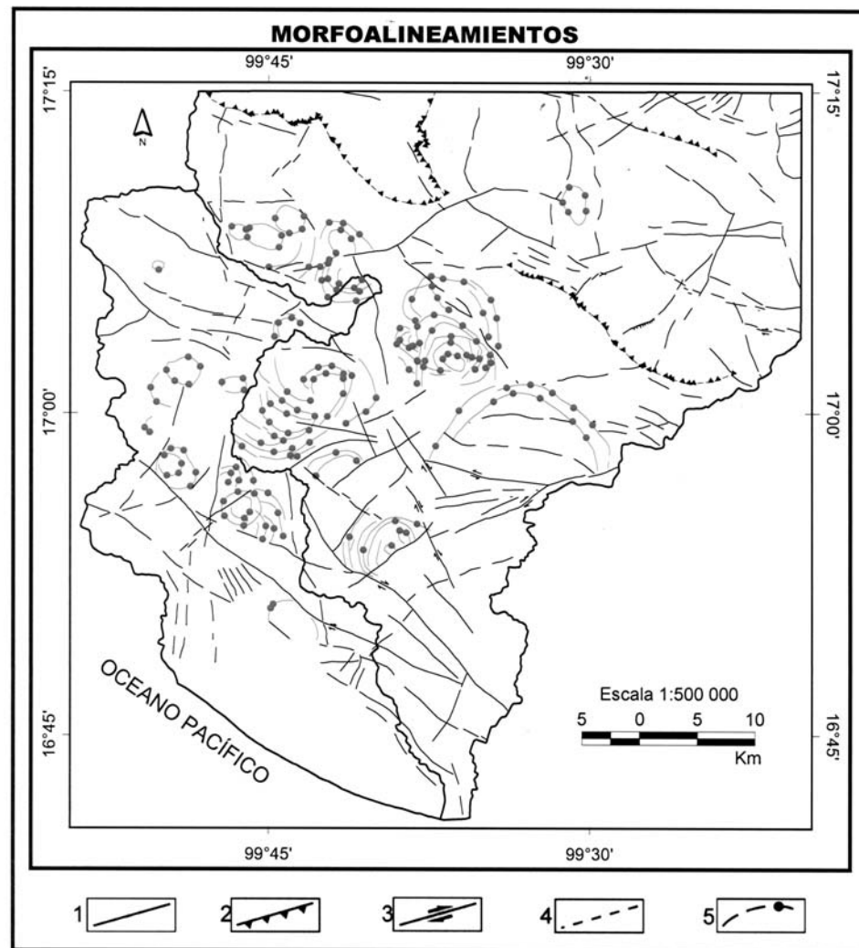
Figura 4. Principales estructuras geológicas del territorio: 1. Fallas por datos geológicos; 2. Fallas inversas; 3. Fallas transcurrentes; 4. Morfoalineamientos; 5. Estructuras circulares.
