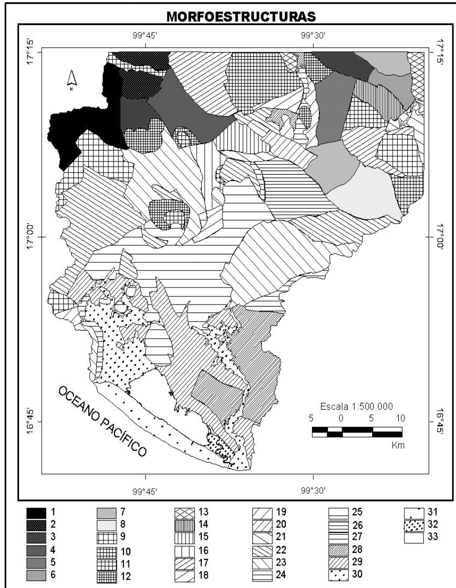
Figura 5. Morfoestructuras de los tercios medio e inferior de la cuenca hidrográfica del río Papagayo y de la cuenca del río Sabana, estado de Guerrero (véase leyenda).
