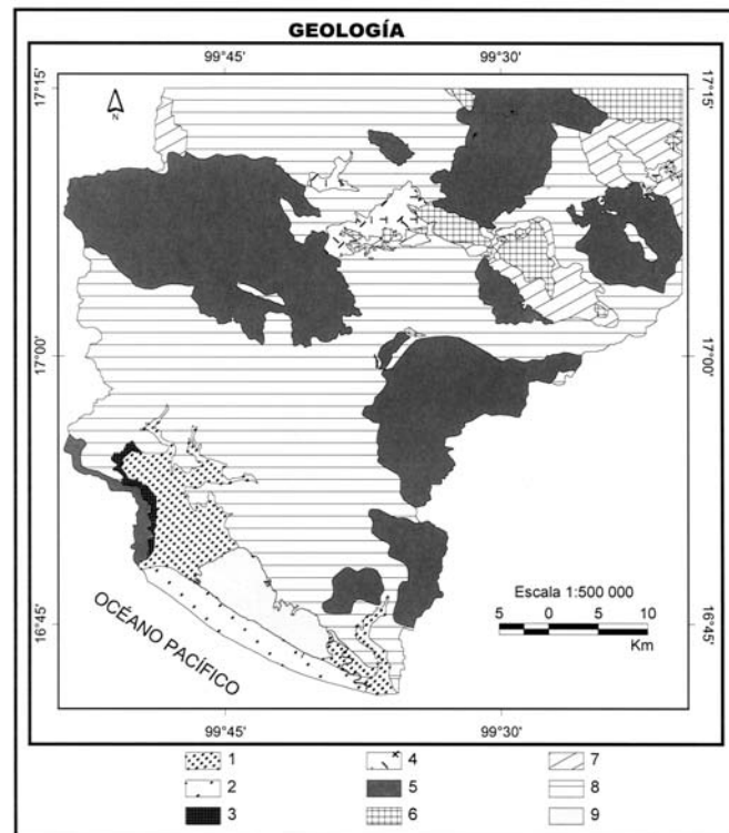
Figura 2. Geología del área de estudio. 1. Aluvión cuaternario de arenas y arcillas; 2. Depósitos arenosos litorales del Cuaternario; 3. Depósitos detríticos, coluvio-proluviales, del Cuaternario; 4. Derrames lávicos con depósitos piroclásticos de composición riolítica de la Formación Papagayo, del Mioceno; 5. Granitos, granodioritas, tonalitas y cuarzo-monzonitas, del Cretácico; 6. Calizas y dolomías, en capas gruesas, de la Formación Morelos, del Cretácico inferior; 7. Areniscas, limolitas, conglomerados, esquistos, pizarras y filitas de la Formación Chapolapa, del Triásico; 8. Gneises cuarzo-feldespáticos y pelíticos, esquistos de biotita, migmatitas y diques ácidos a básicos del complejo Xolapa, del Paleozoico; 9. Laguna de Tres Palos.
