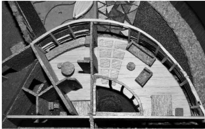
Fotografía 5. Vista superior de la vivienda con mobiliario removible. Se aprecia sala/comedor, cocina, jardín interior y servicios higiénicos.
