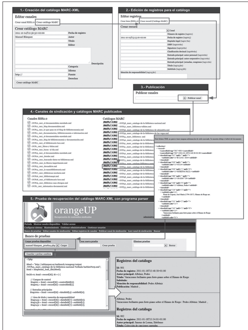
Figura 1. Cadena de procesos en la edición y publicación de catálogos bibliográficos: http://www.mblazquez.es/documents/orangeup-process.png
