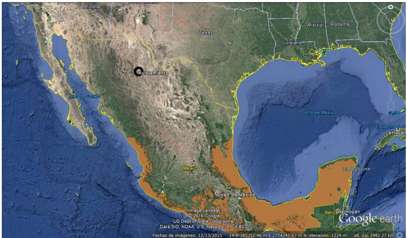
Figura 1. Distribución de estancia neotropical de Setophaga dominica (chipe garganta-amarilla) en color naranja; distribución potencial reportada por Navarro y Peterson (2007); el círculo negro, en Chihuahua, es el presente registro.
