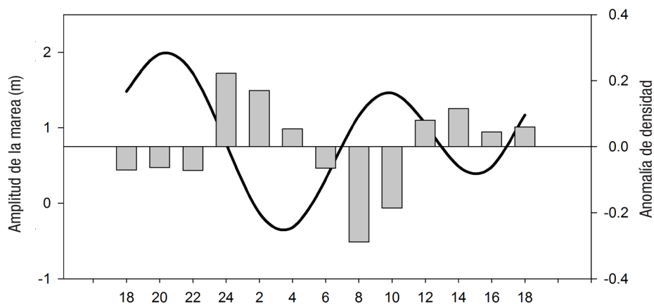
Figura 7. Variación diaria de la amplitud de marea y diferencias de densidad en la capa a 30 \text{ m} medidos en la boca de Bahía Magdalena, México. Los valores positivos corresponden al reflujo y los negativos al flujo.
