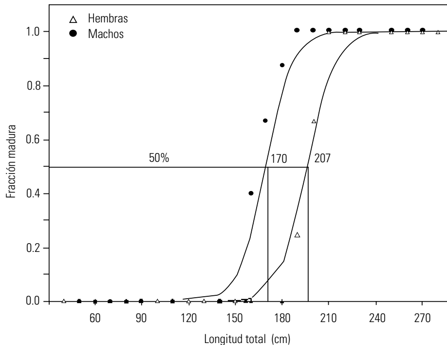
Figura 6. Relación entre la madurez y la longitud total de machos ( n = 24 ) y hembras ( n = 28 ) de S. lewini . Las líneas representan el modelo logístico ajustado por la técnica de máxima verosimilitud.
