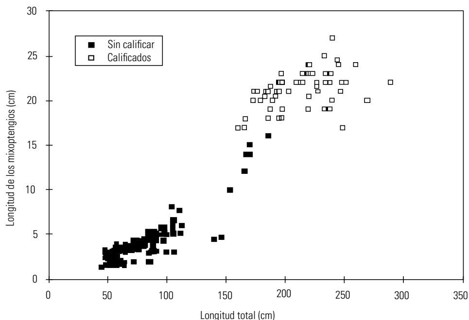
Figura 5. Relación entre la longitud total y la longitud de los mixopterigios de machos de S. lewini capturados en el Golfo de California ( n = 311 ).
